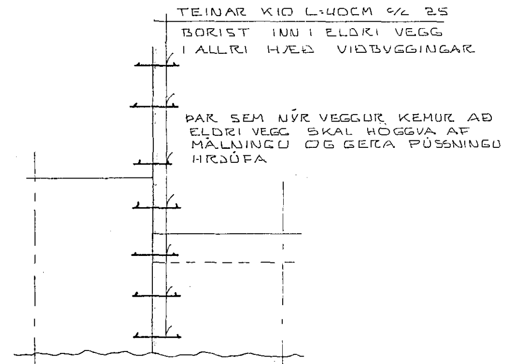
ÚTLIT D-D 1:20
