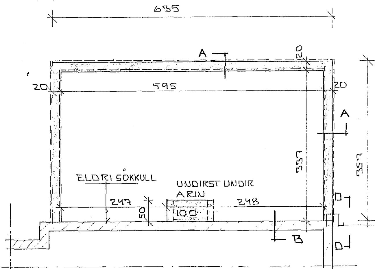
GRUNNMYND UNDIRSTÖÐUR M 1:50
