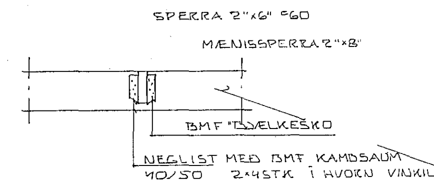
SNID E 1:20
