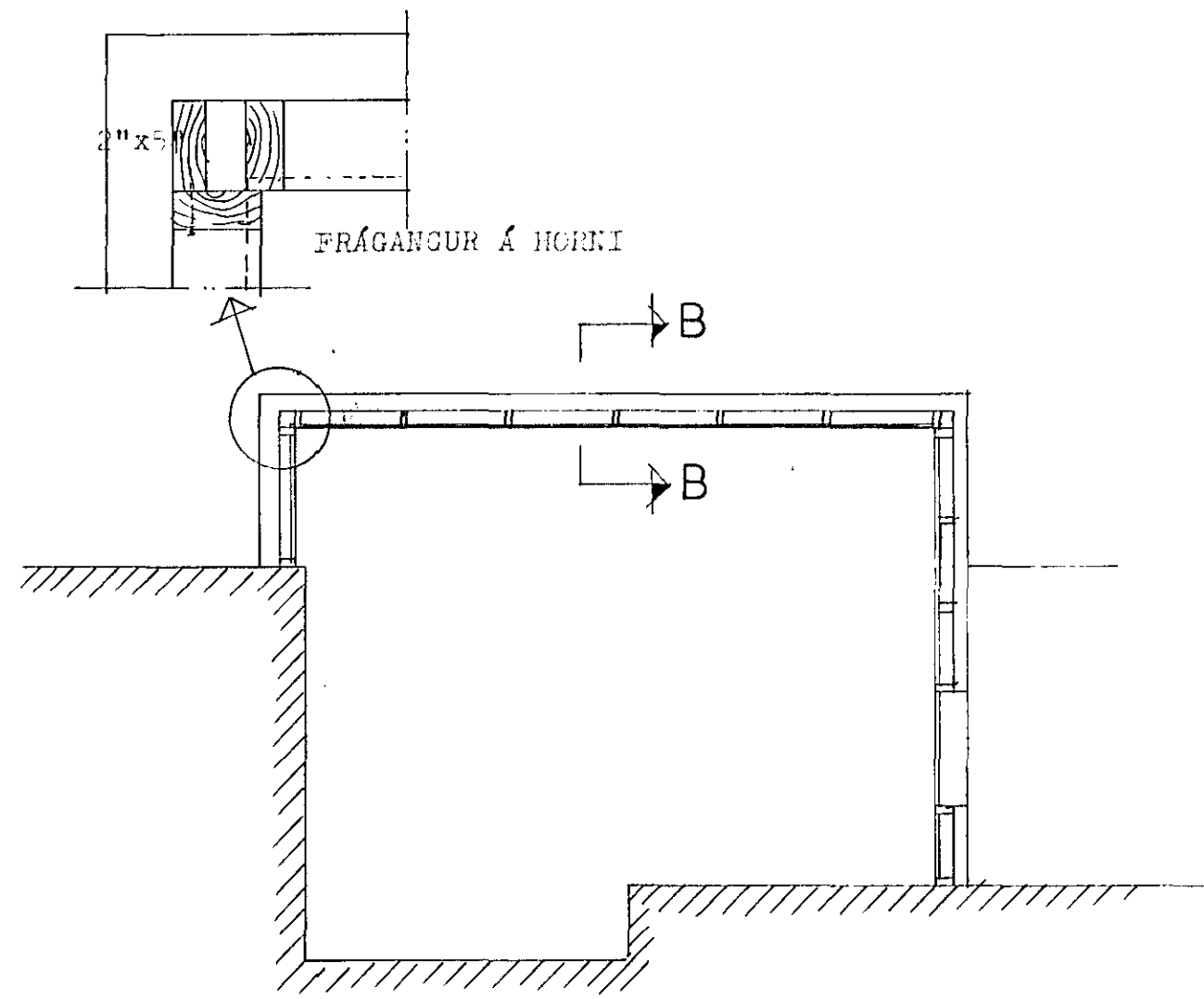
GRUNNMYND 150
