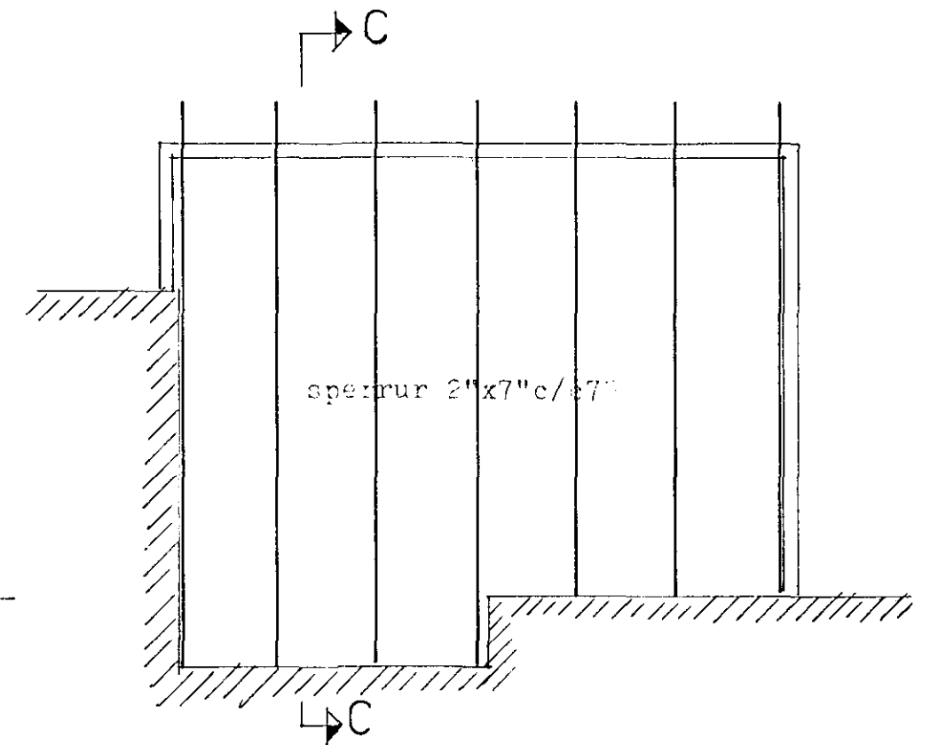
GRUNNMYND 150
