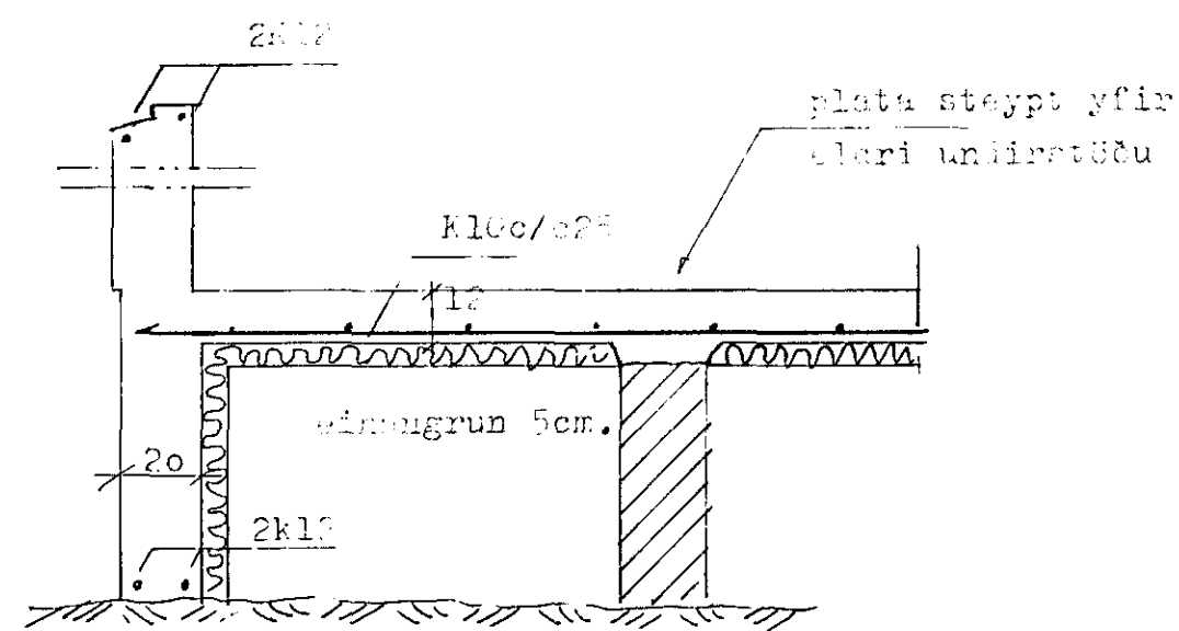
SNID A-A 1:20
