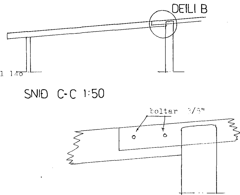
DEILI B 1:20
