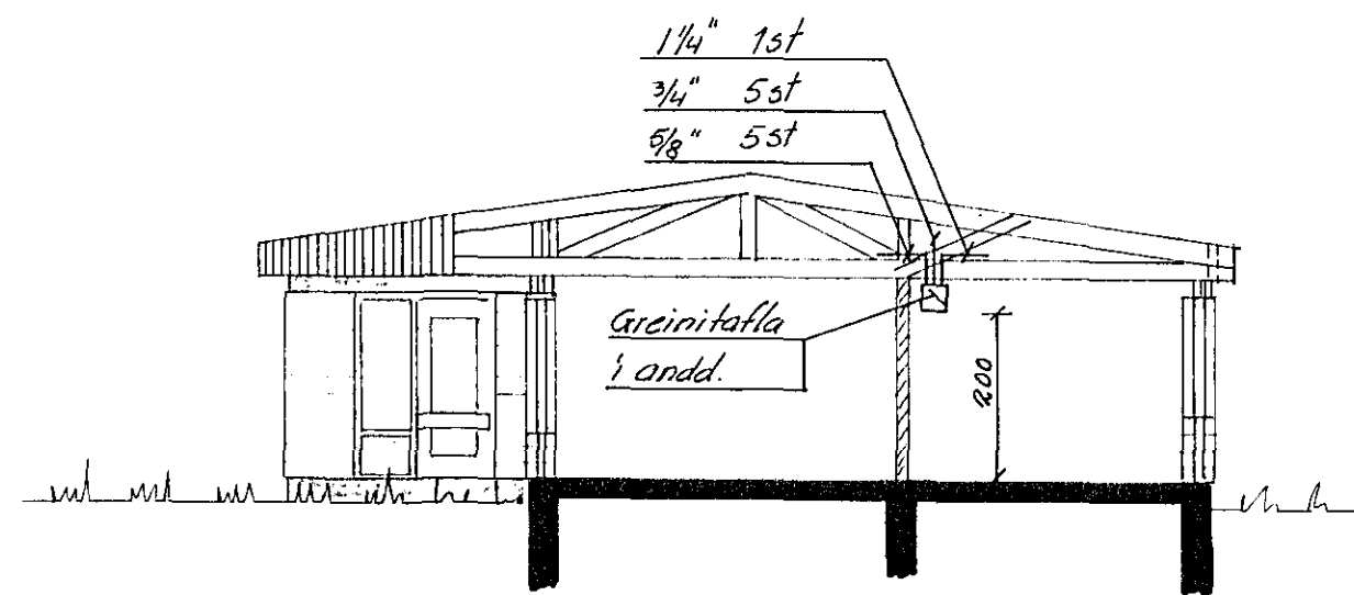
A-A
