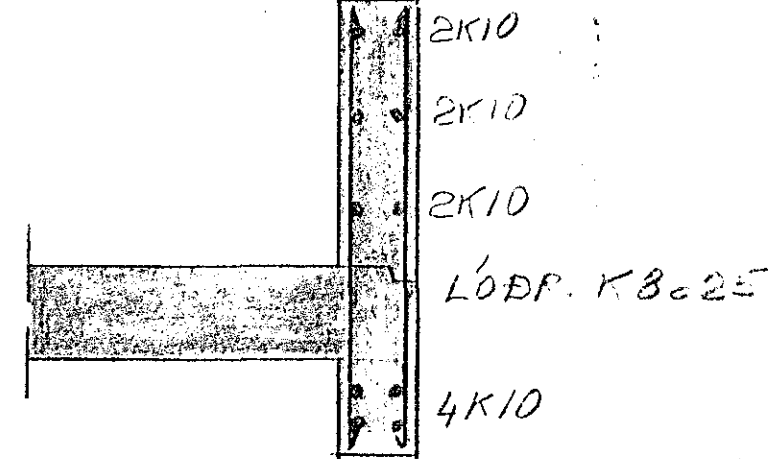
AB 1:20
