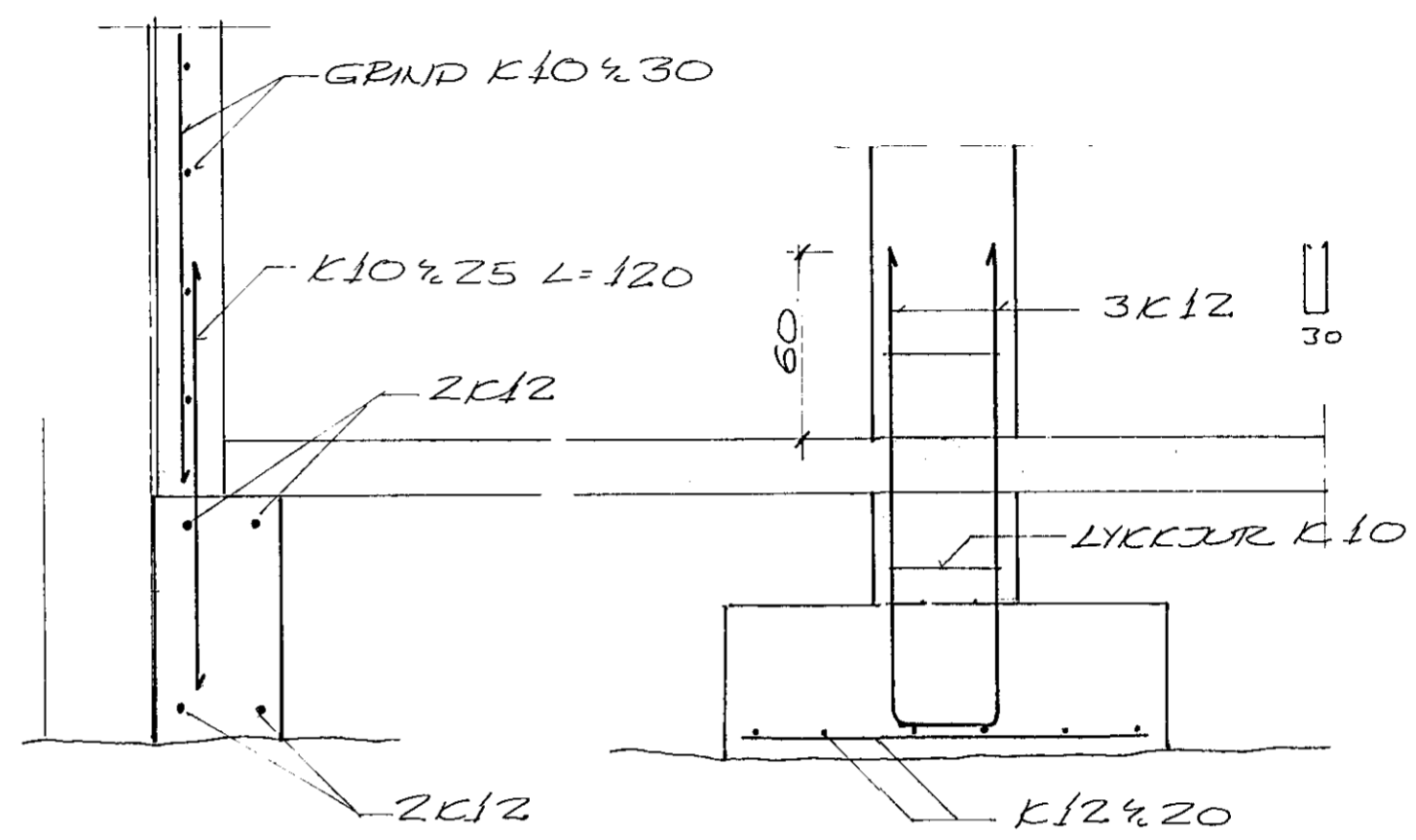
SNID A-A 1:20
