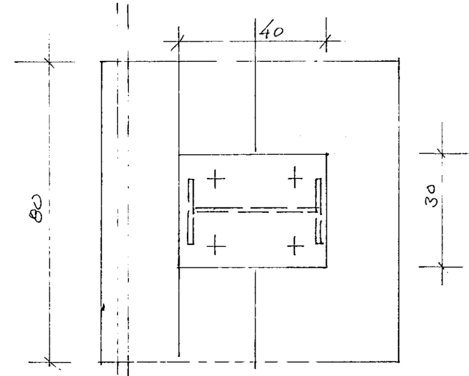
UNDIRSTÖÐUR 1:10
