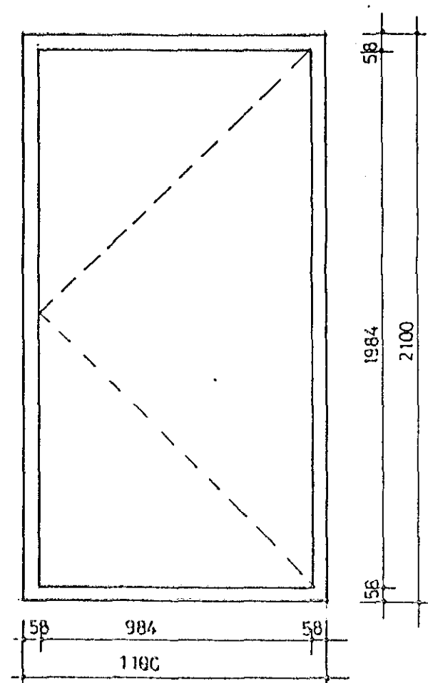
HURÐ FYRIR GEYMSLU, 1:20
