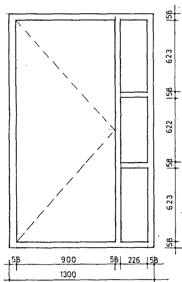
HURÐ FYRIR FÖRSTOFU, 1:20
