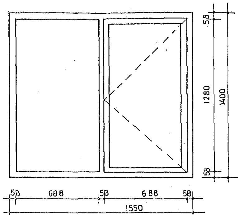
GLUGGI G1, 1:20 10 STK OG 2 STK. SPEGILMYND.
