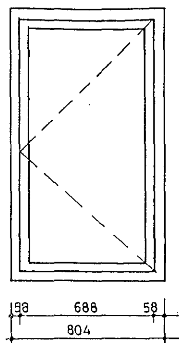
GLUGGI G2, 1:20 4 STK.
