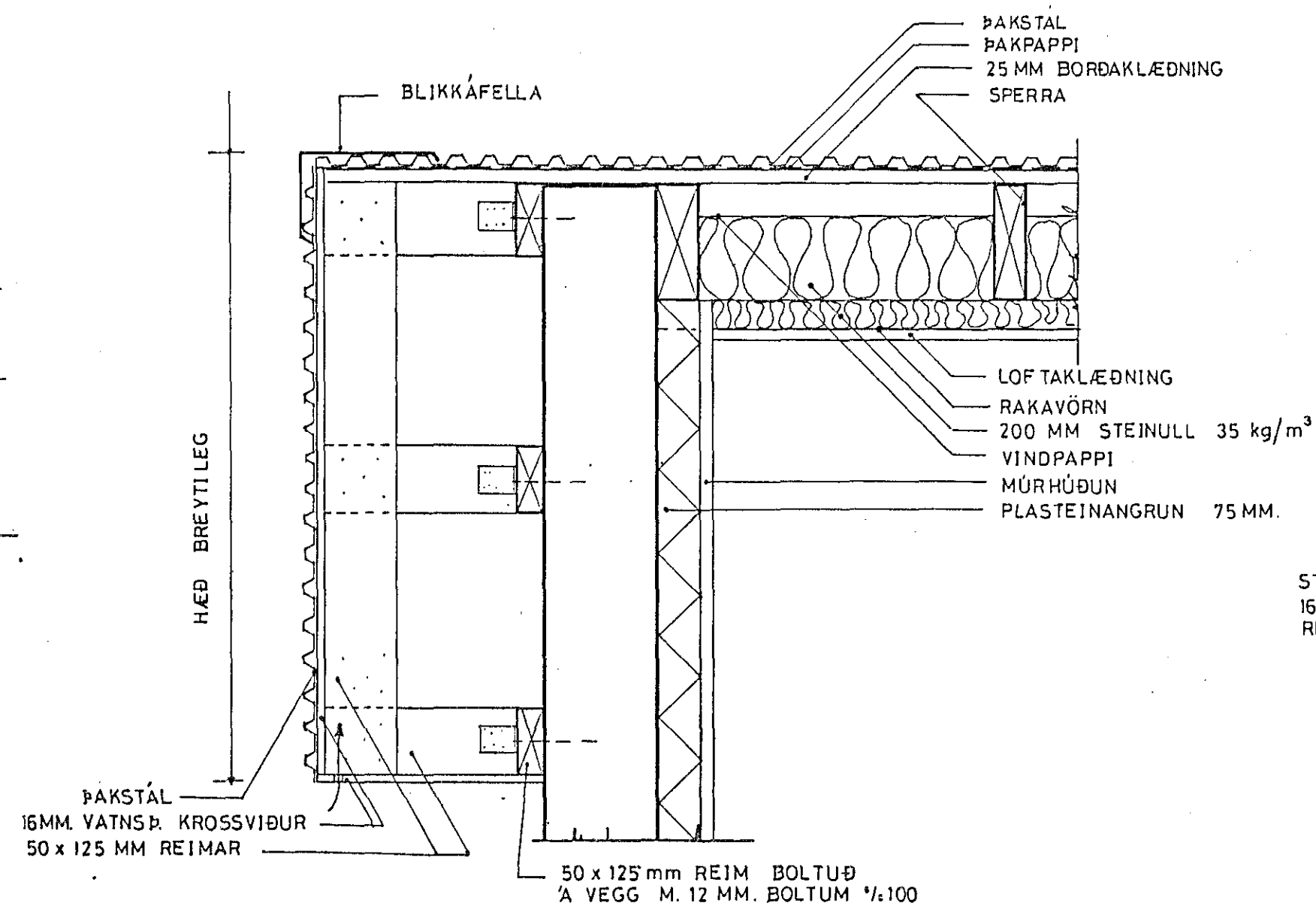
FRÁGANGUR Á STÖFNUM, 1:10
