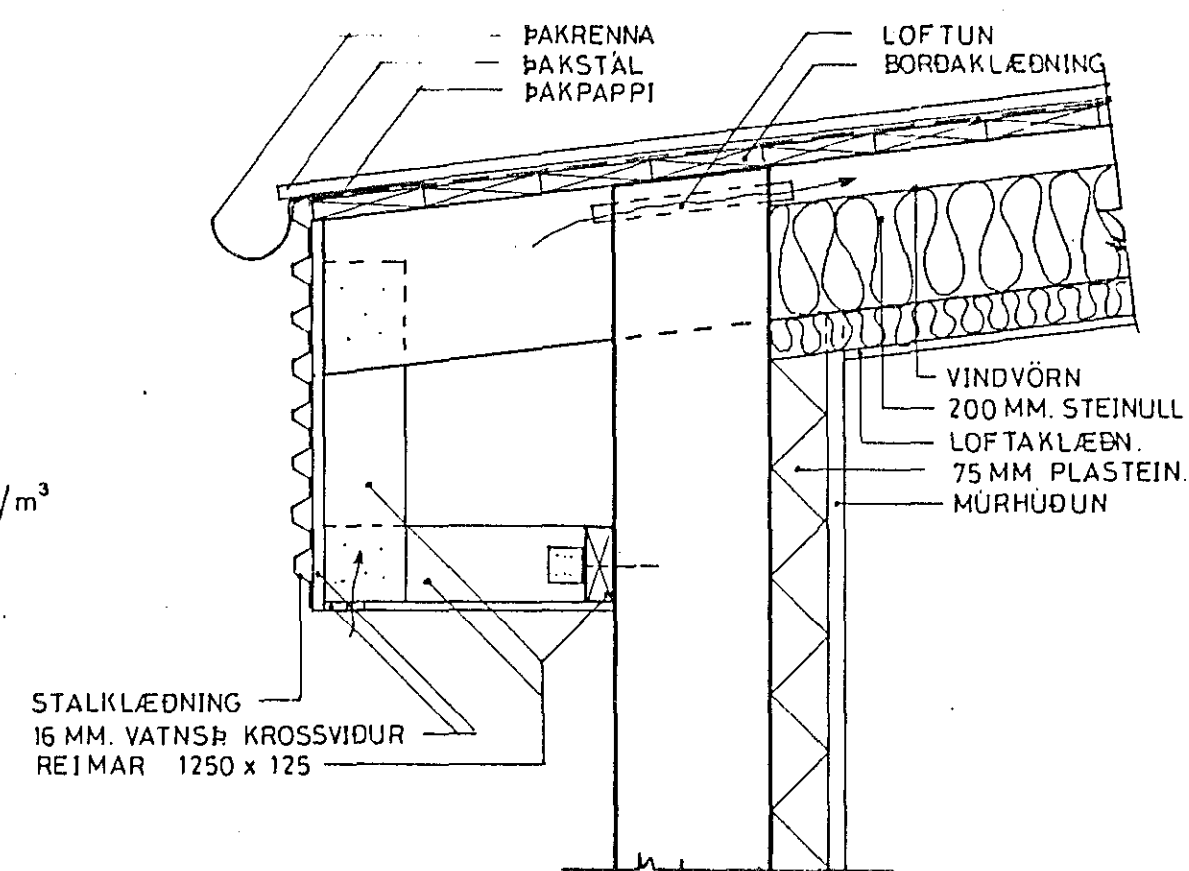
FRÁGANGUR Á ÞAKBRÚN, 1:10
