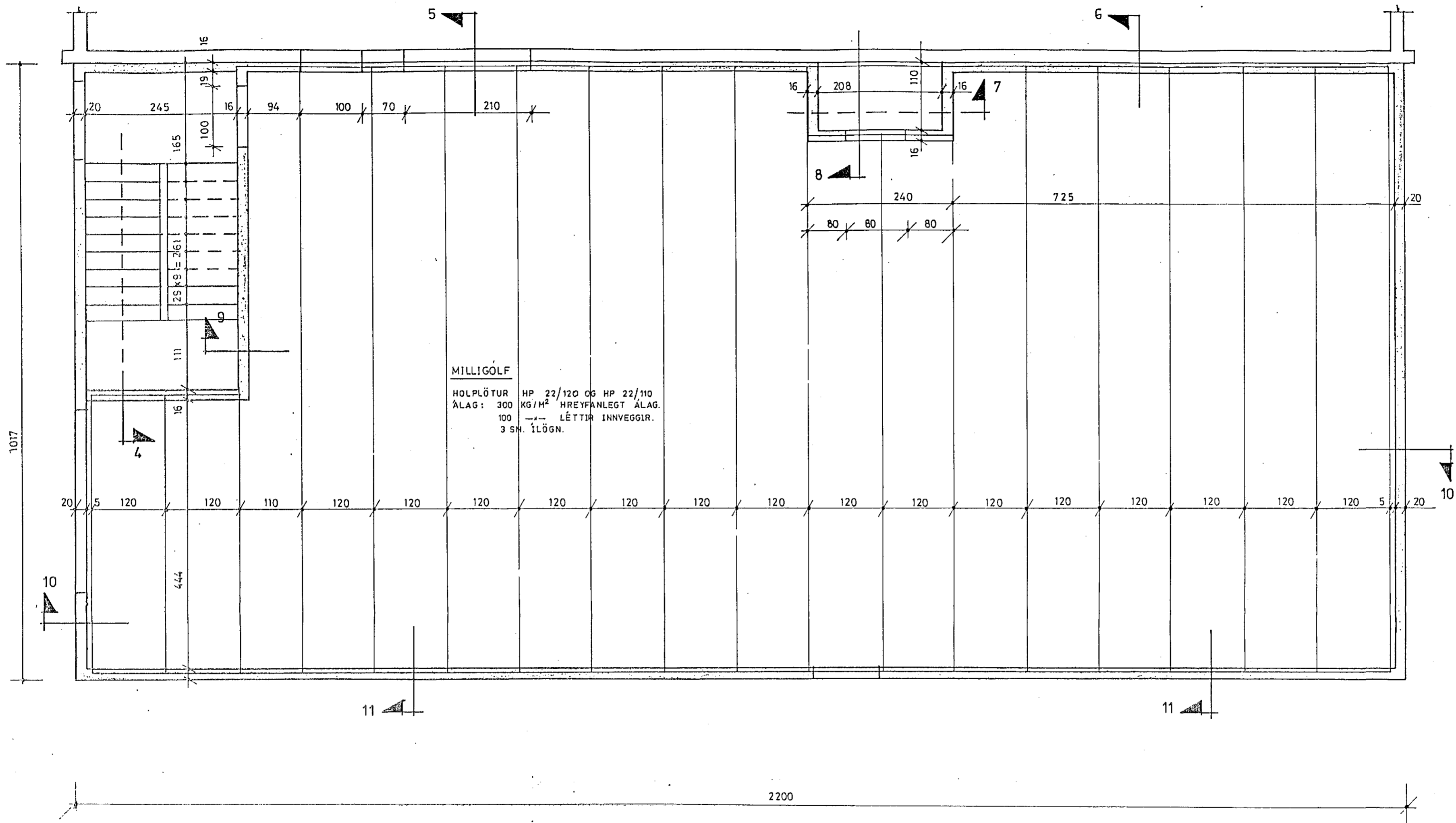
GRUNNM. 1.H. - MILLIGOLF 1:50
