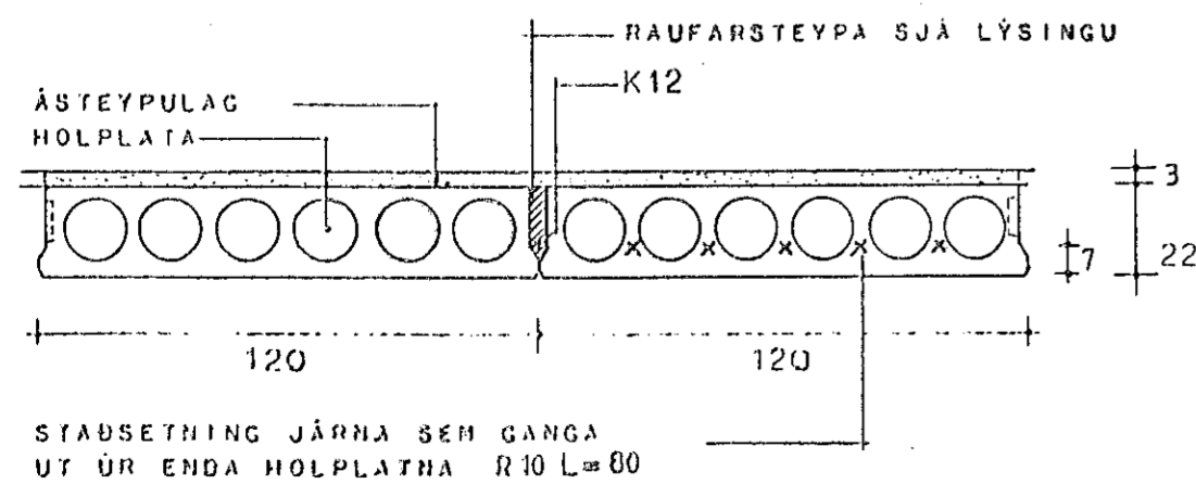
SAMSETNING HOLPLATNA 1:20
