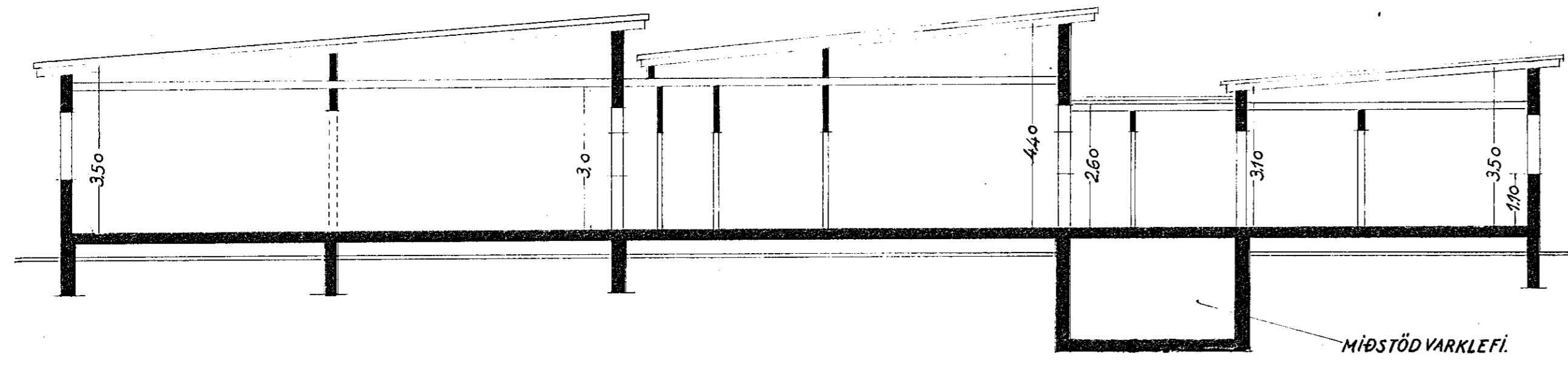
Sneiðing.
