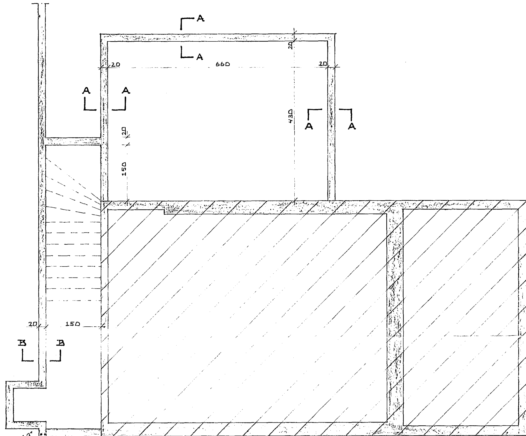
GRUNNMYND 1:50
