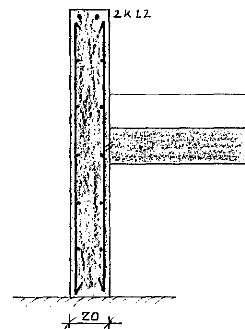
SNIB D-D 1:20
