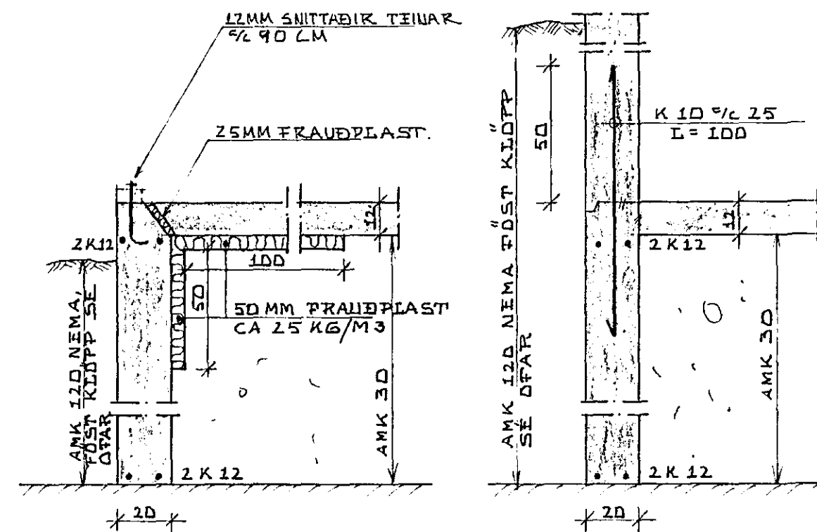
SNIB A-A 1:20
