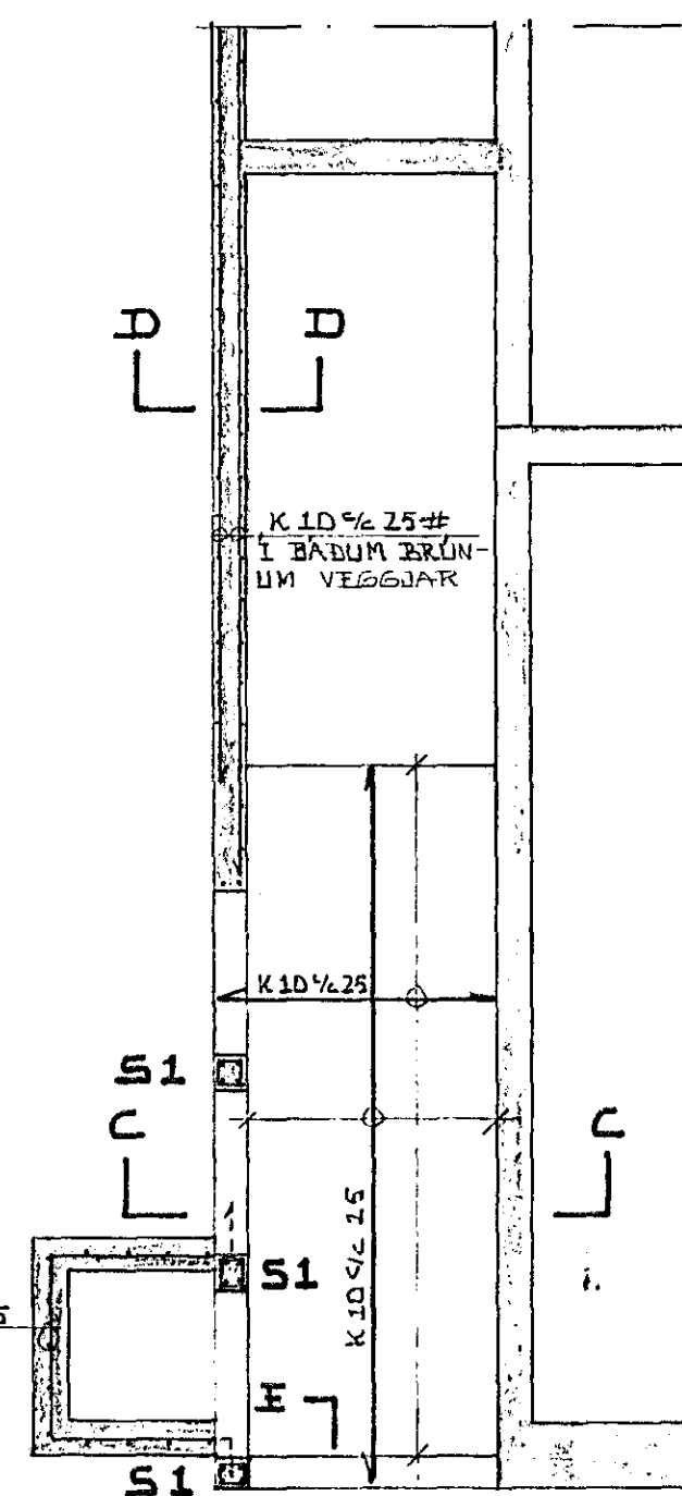
GRUNNMYND UNDIRGANGS 1:50
