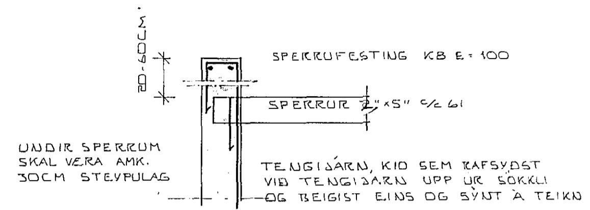
SPERRUFESTING 1:20
