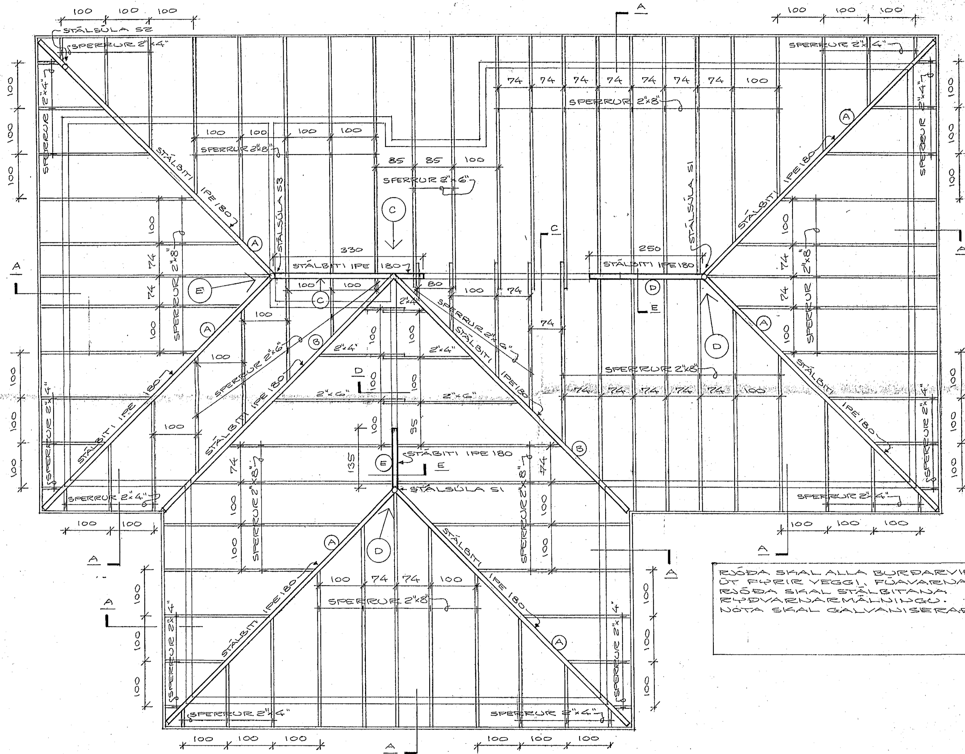
GRUNDMYND, M=1:50
