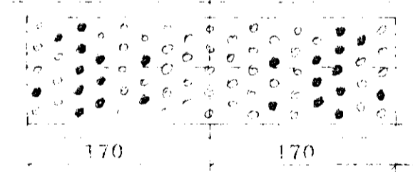
BMF gataplata 340x100x1,5 beggja vegna. Kambsaumur 2x12 stk. 10x10 pr. plötu.
