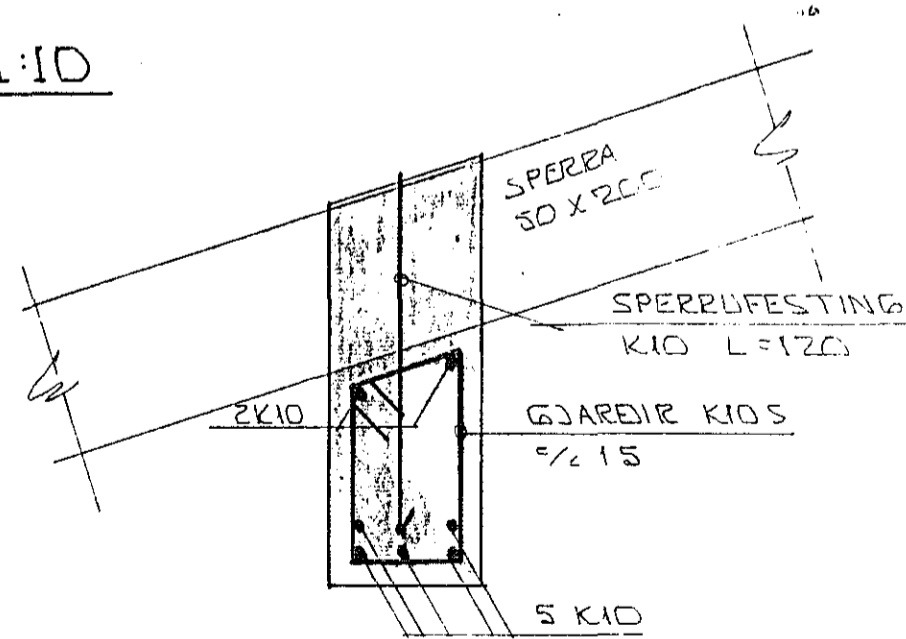
SNID A I BITA - 1:10
