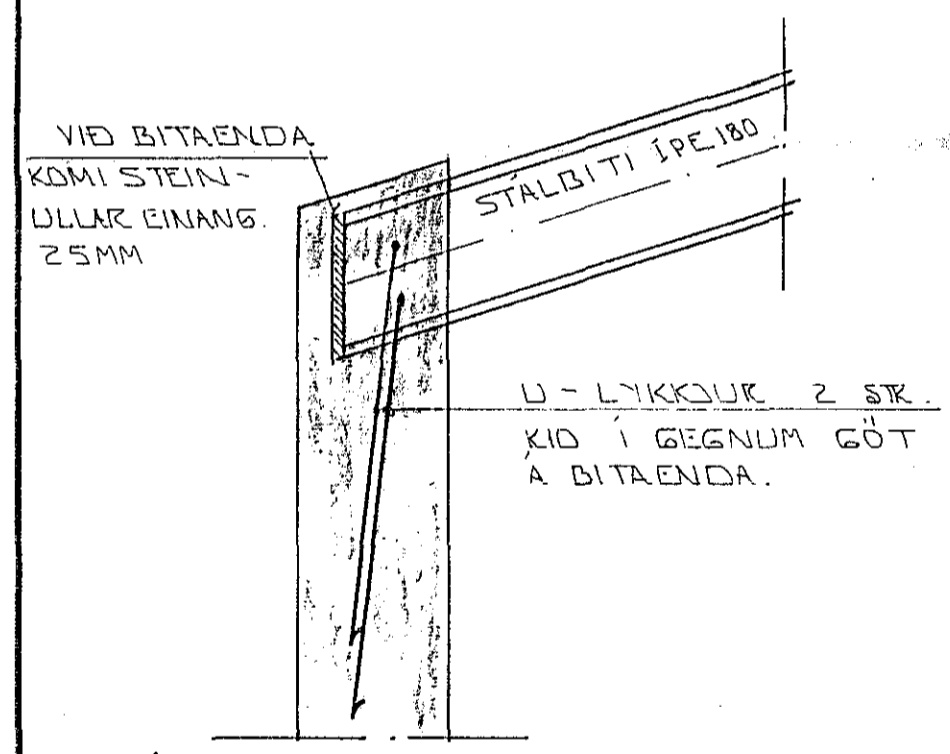
FRÁGANGUR STALBITA Í VEGG 1:10
