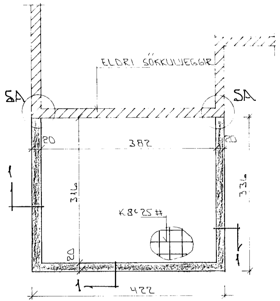
GRUNNMYND 1:50
