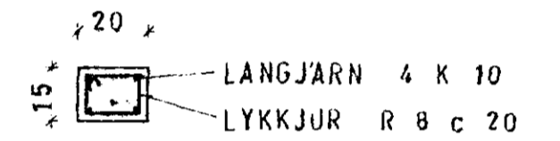
SÚLA S 1 1:20
