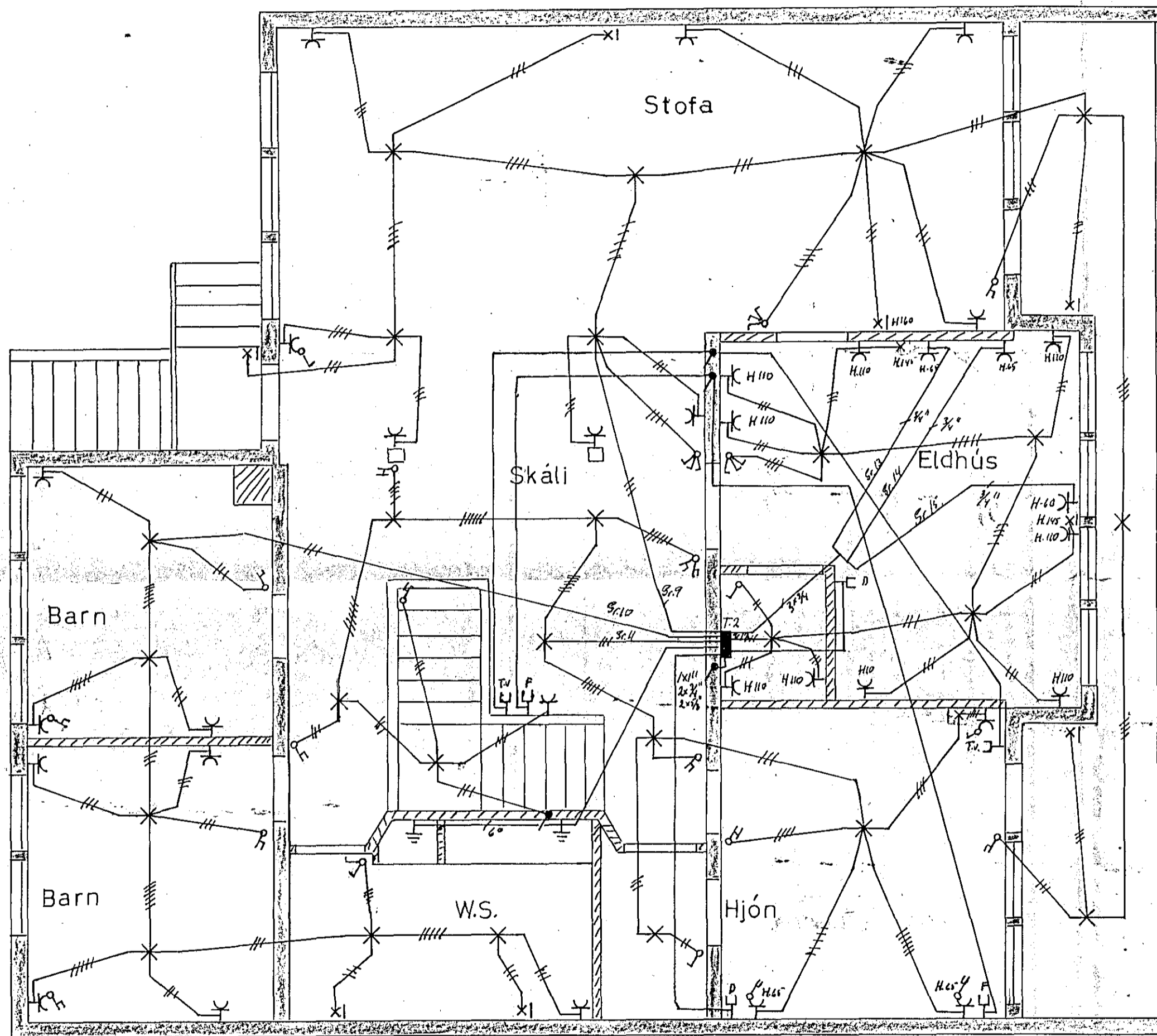
Grúnmynd 2 Hæð 1:50
