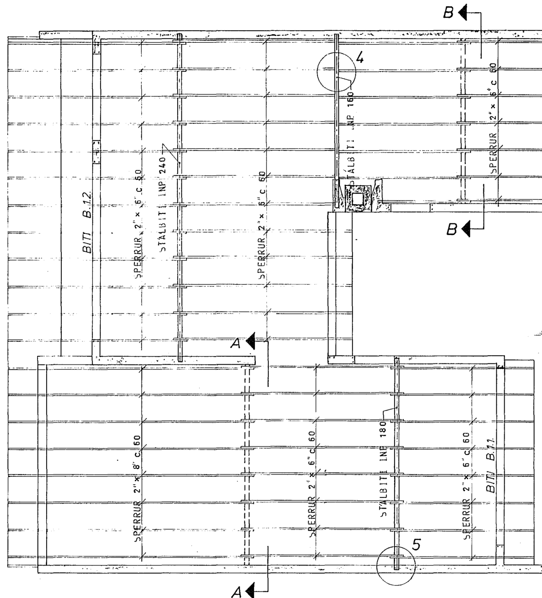
GRUNNMYND - RIS 1:50
