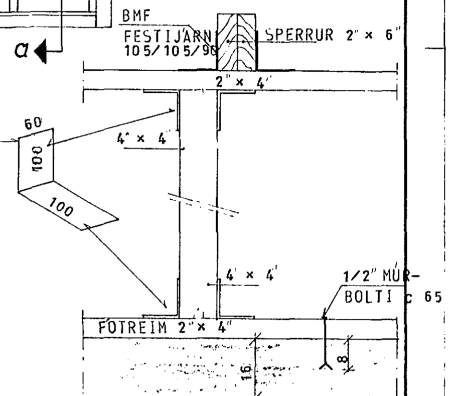
SNID a-a 1:10
