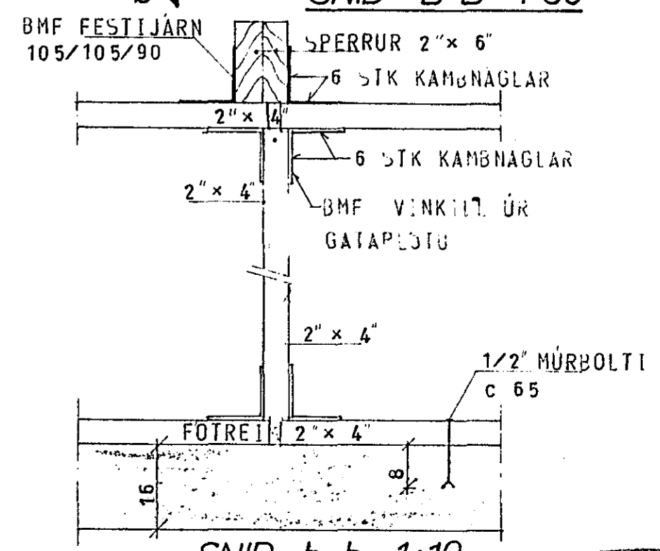
SNID b-b 1:10
