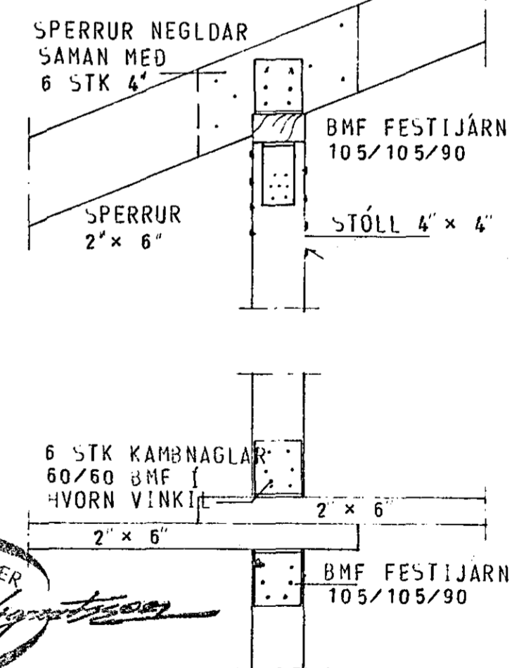
SNID a-a 1:10
