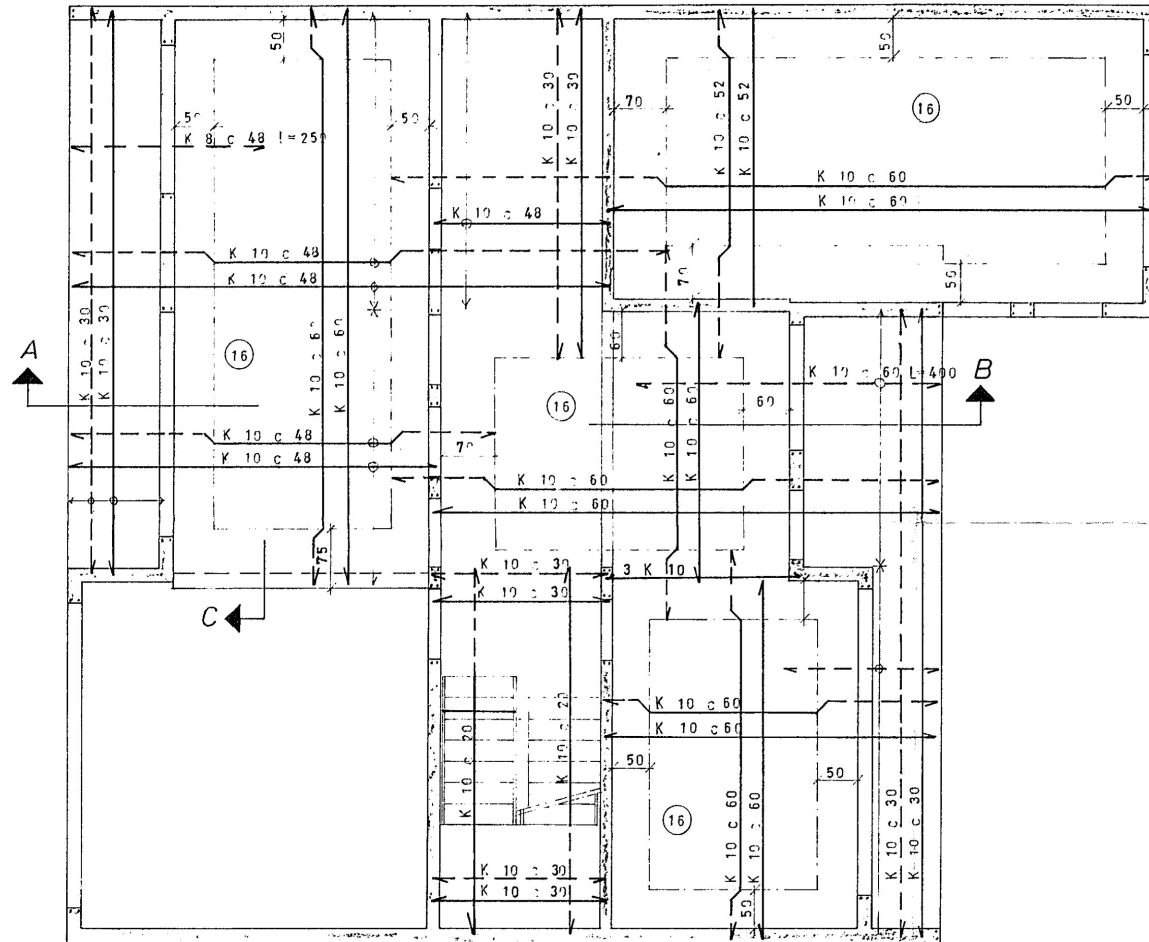
GRUNNMYND — HÆÐAR 1:50
