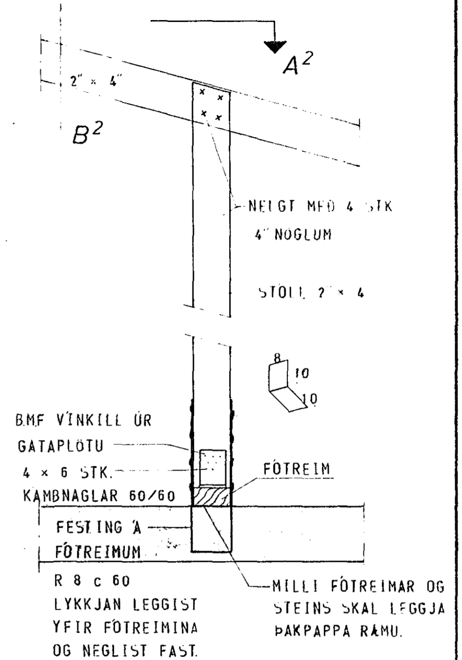
SERMYND 2
