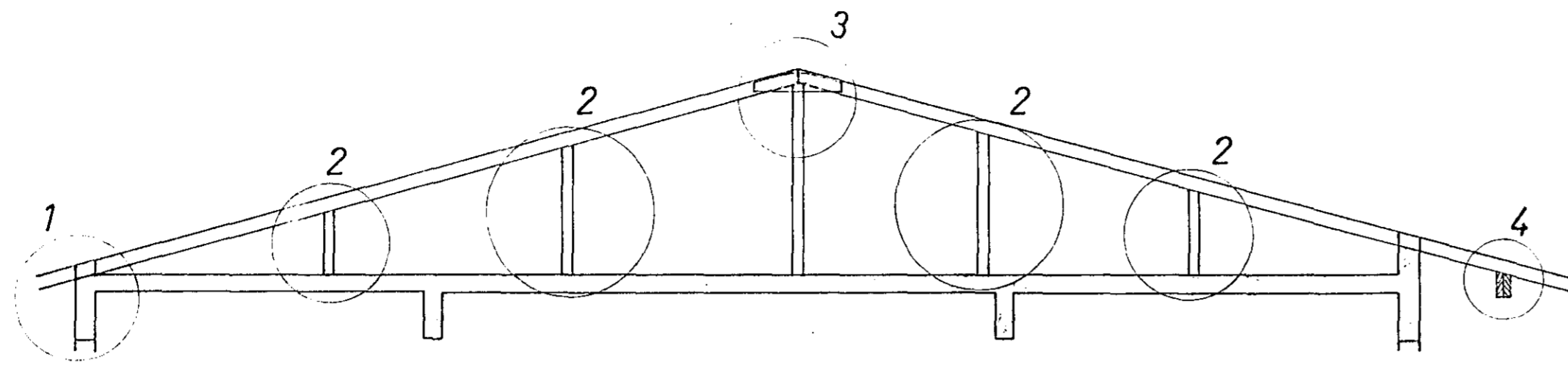
SNID 1 ÞAK 1:50
