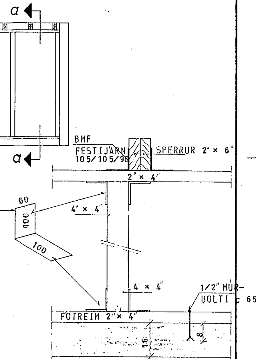
SNID a-a 1:10
