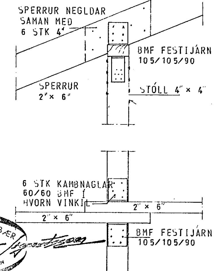
SNID a-a 1:10
