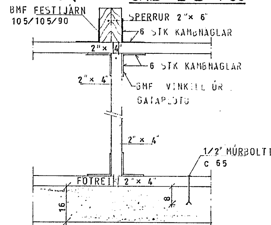
SNID b-b 1:10
