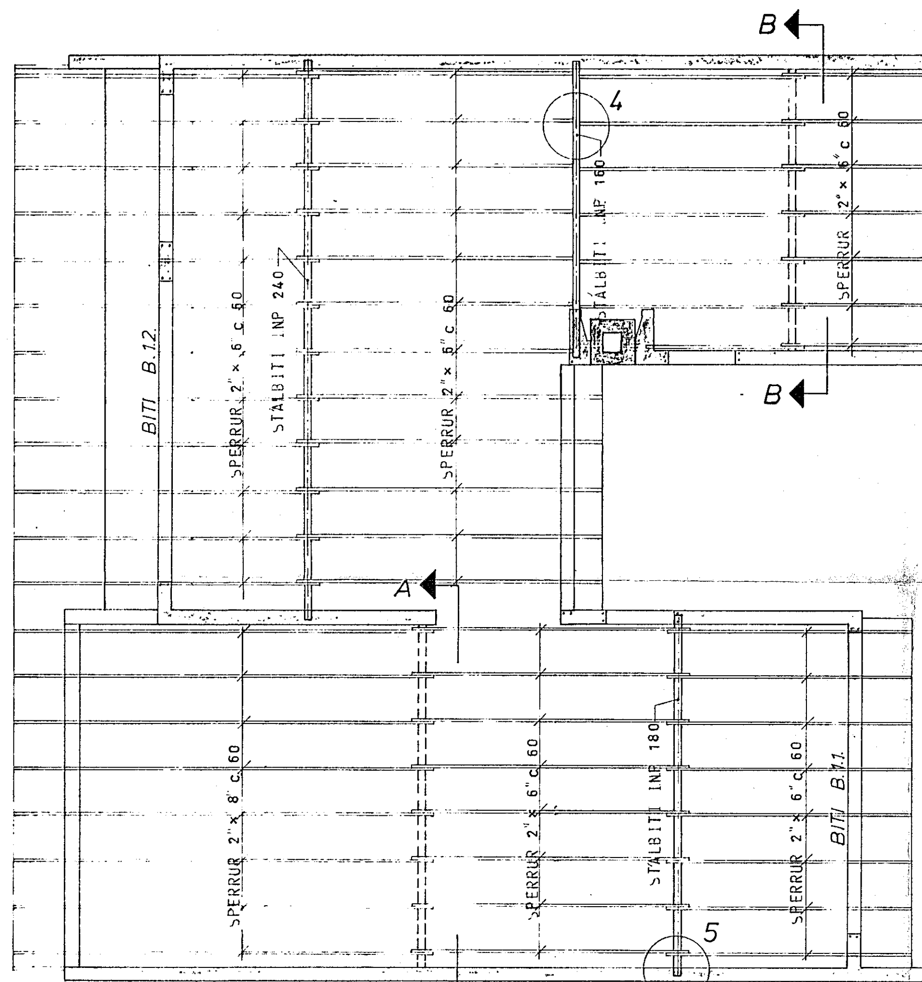
GRUNNMYND - RIS 1:50
