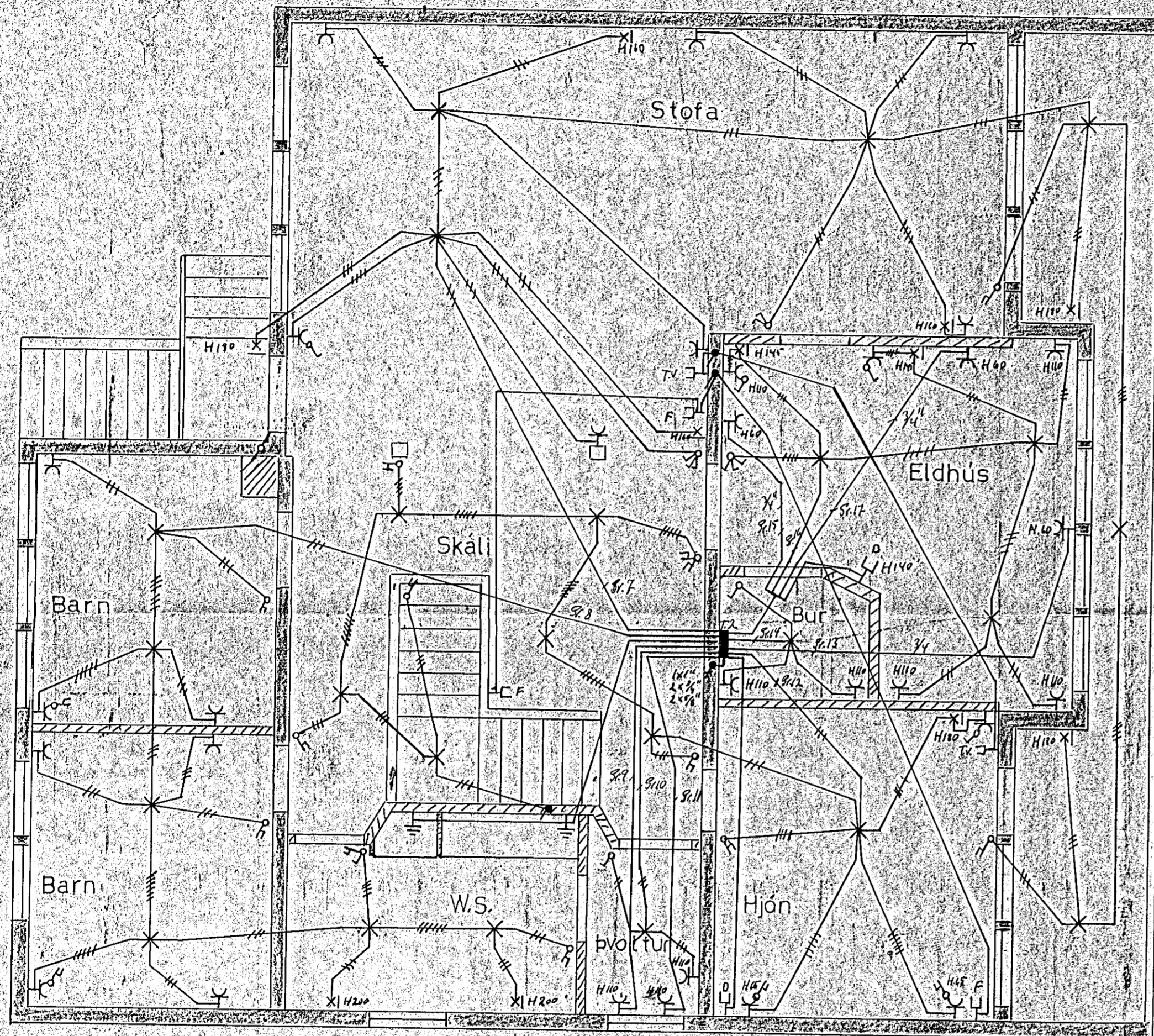
Grunnmynd, 2. hæð 1:50
