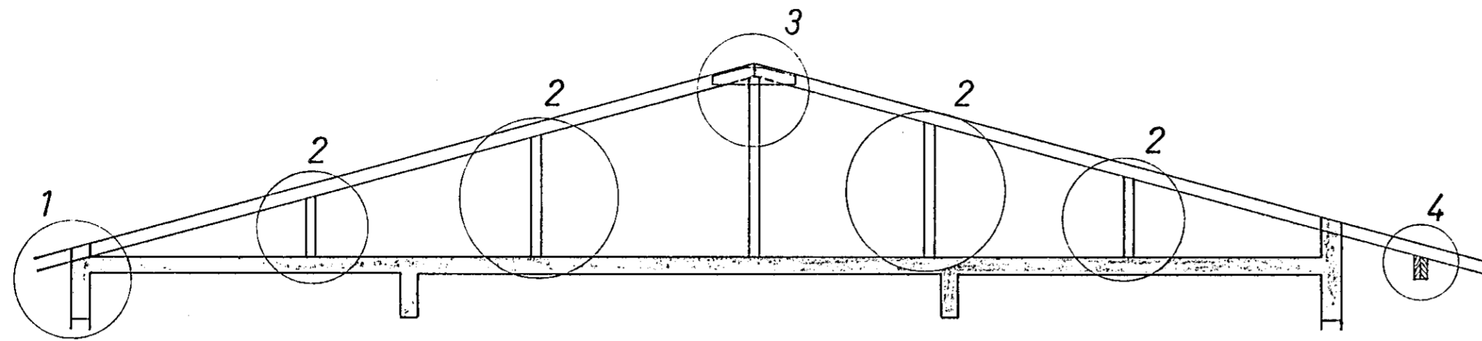
SNID 1 ÞAK 1:50
