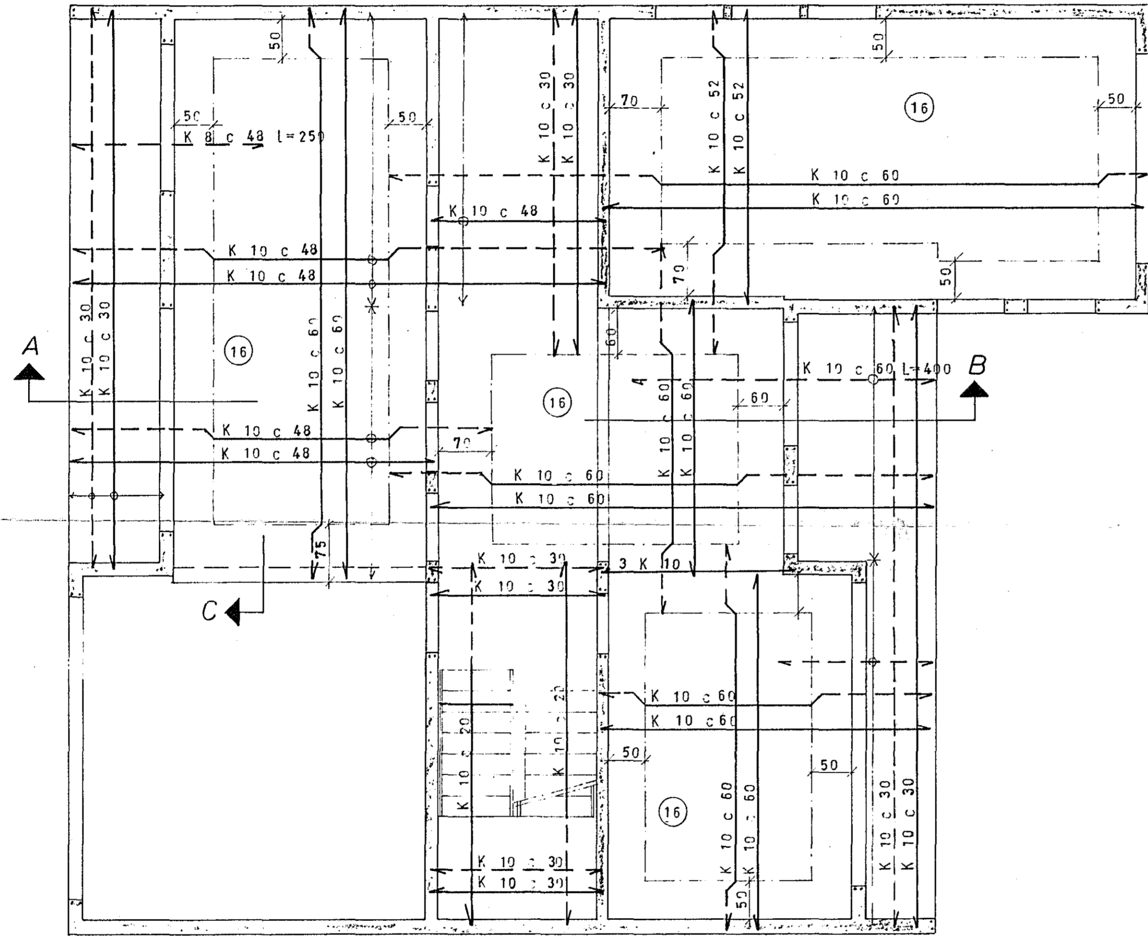
GRUNNMYND — HÆÐAR 1:50
