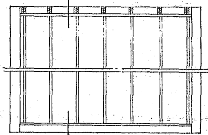
SNID B-B 1:50
