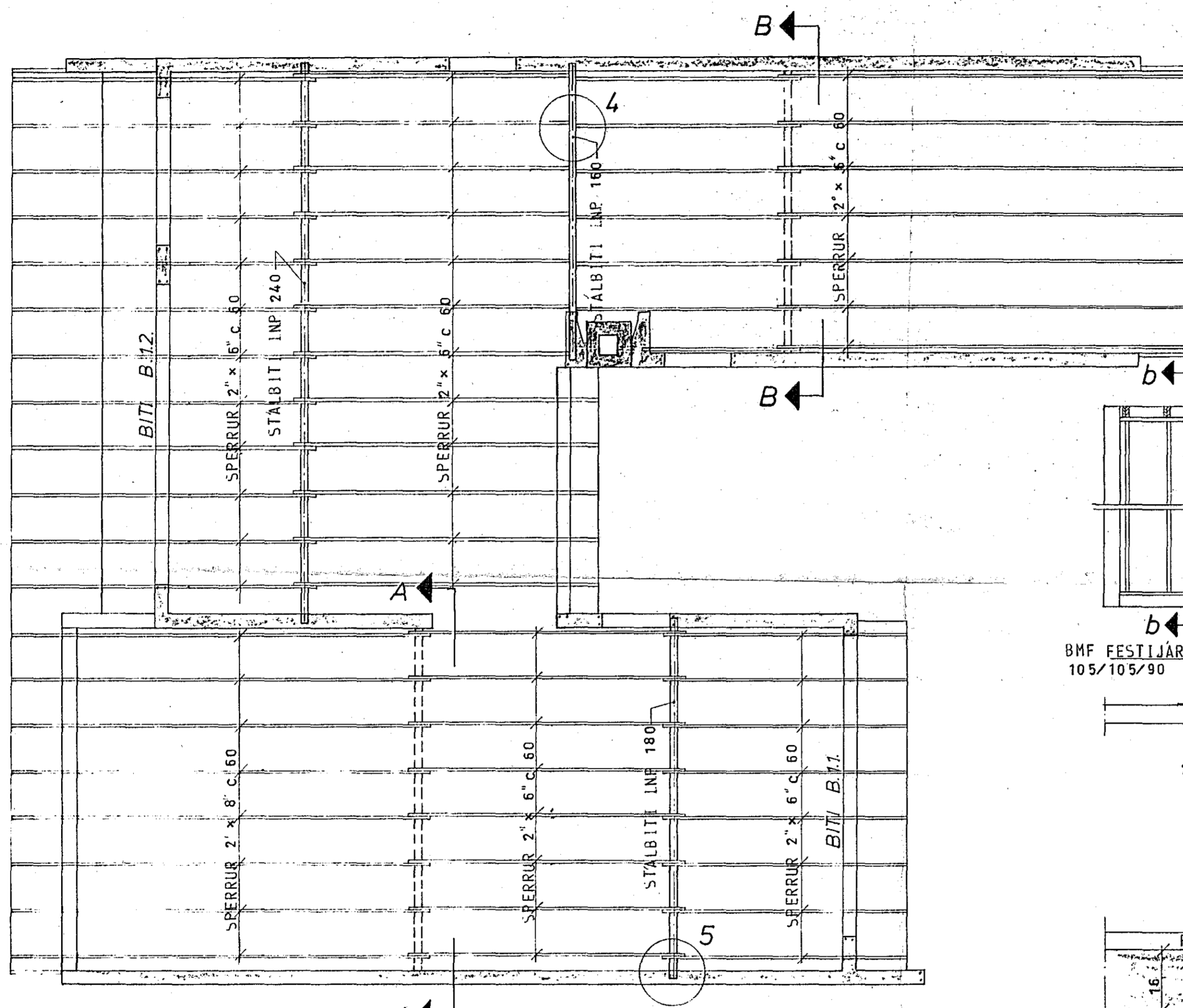
GRUNNMYND - RIS 1:50
