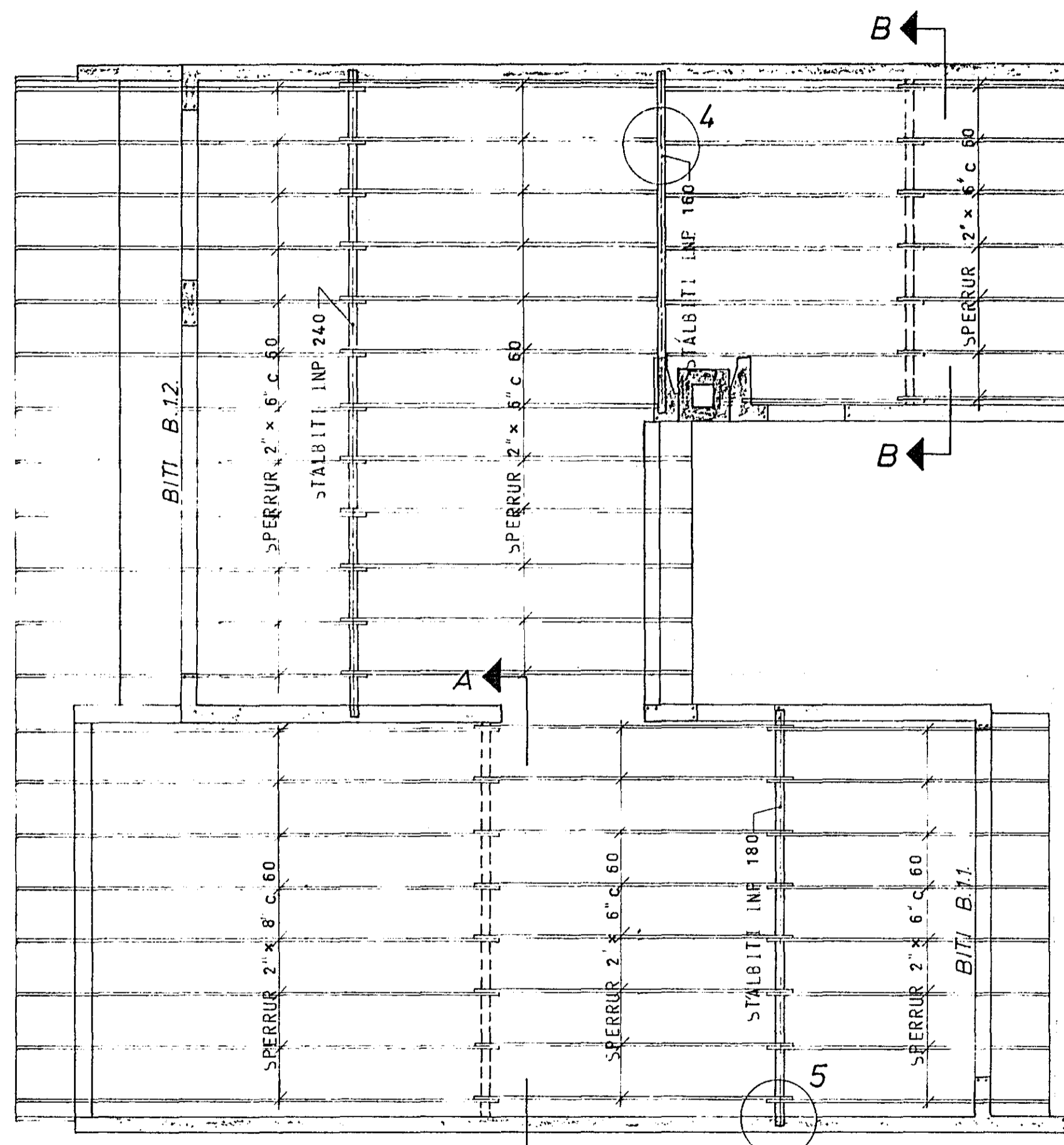
GRUNNMYND - RIS 1:50
