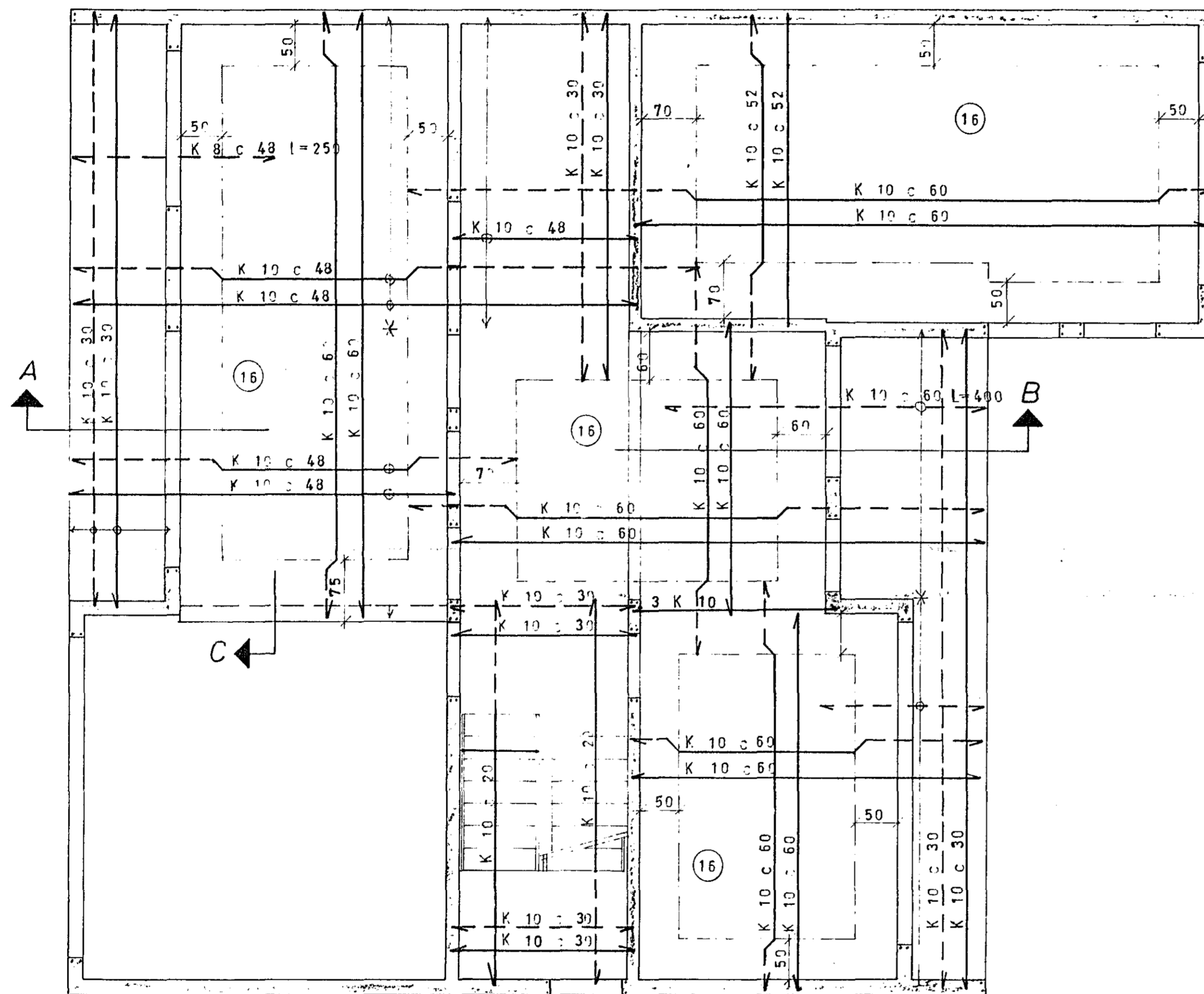
GRUNNMYND — HÆÐAR 1:50
