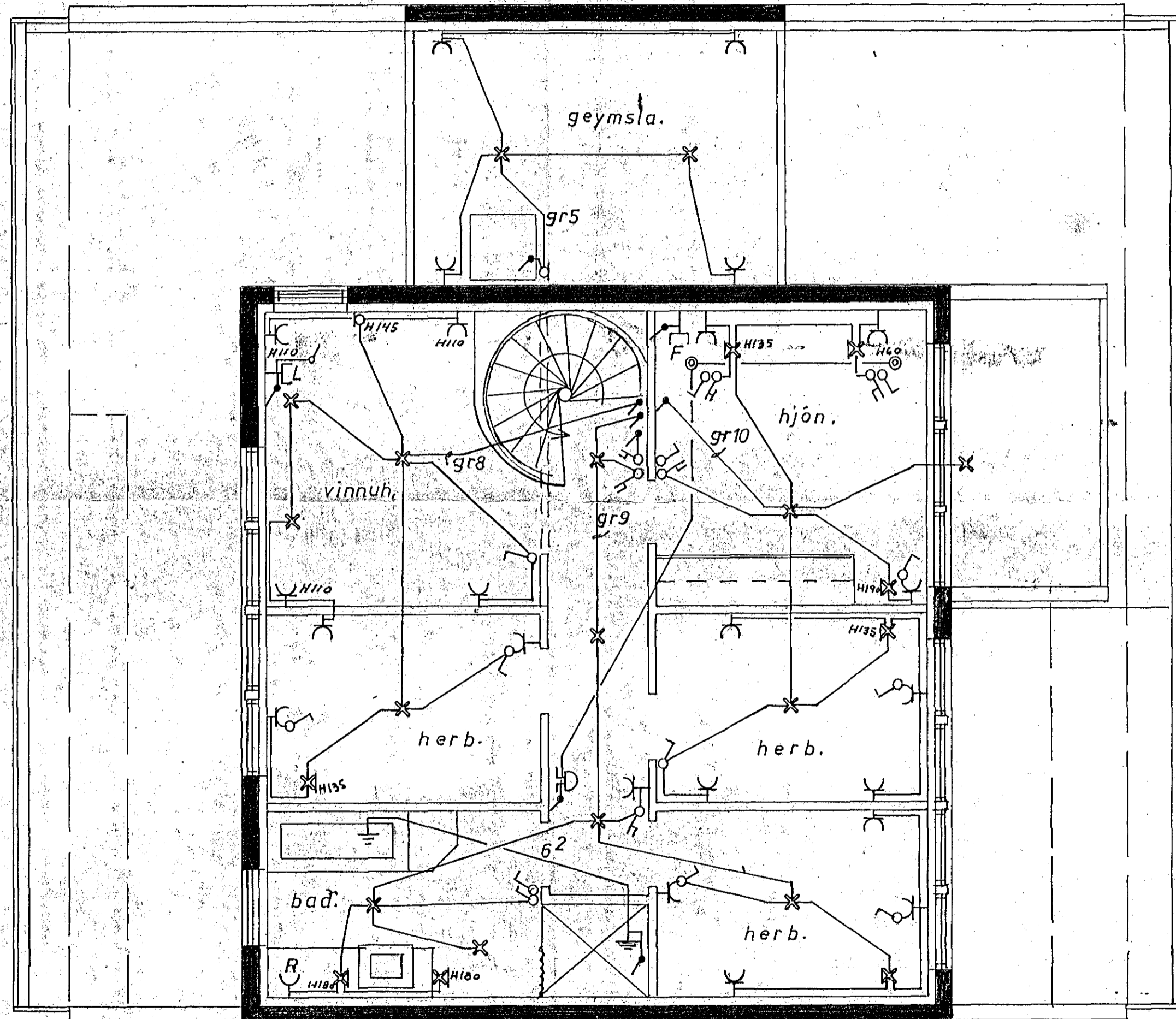
2 HÆÐ. GRUNNMYND MÁL-1:50.
