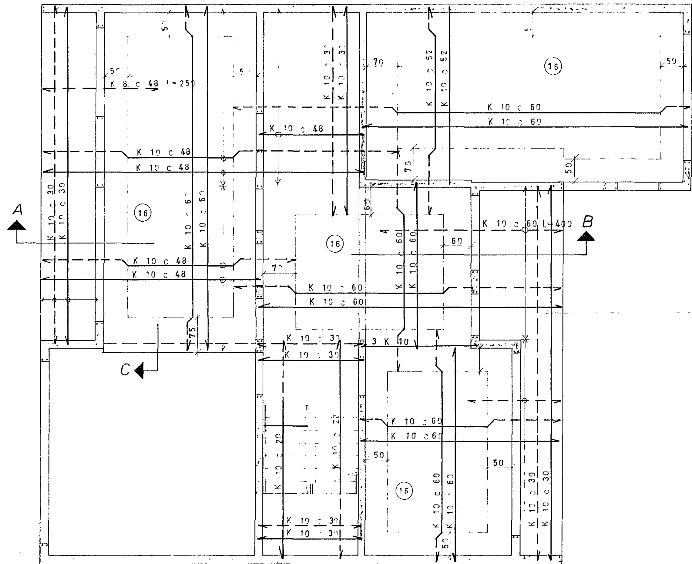
GRUNNMYND — HÆÐAR 1:50
