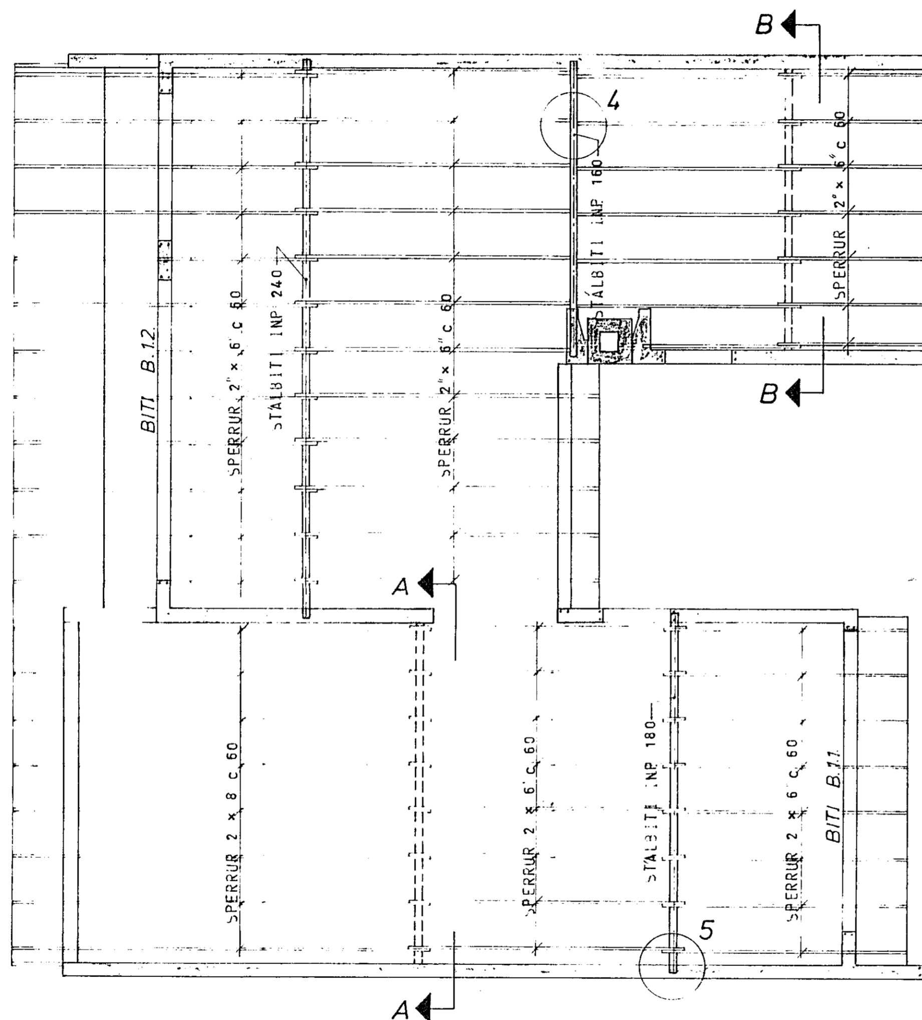
GRUNNMYND - RIS 1:50
