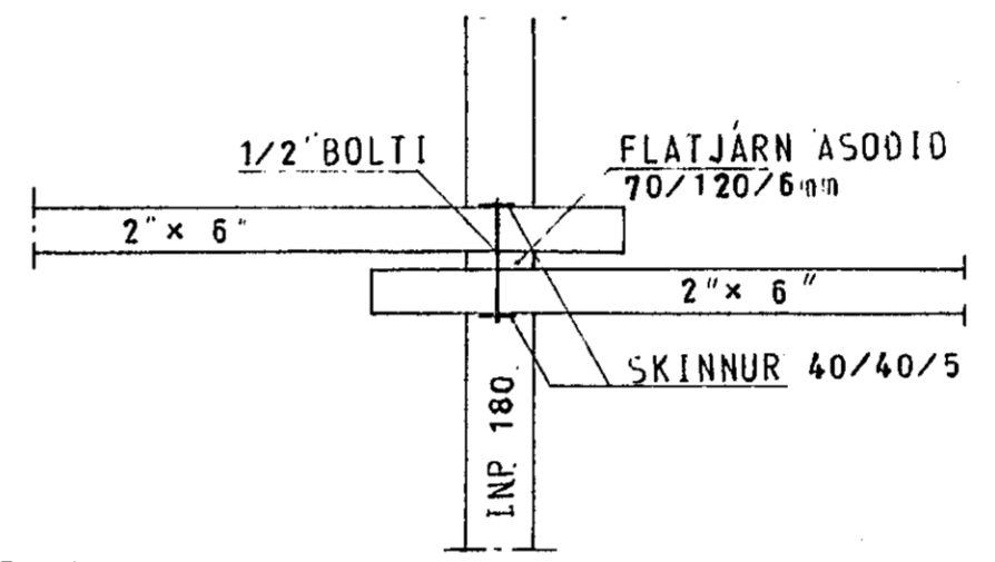
SÉRMÝND 1 1:10
