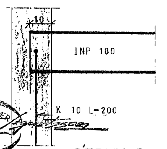
SÉRMÝND 5 1:10
