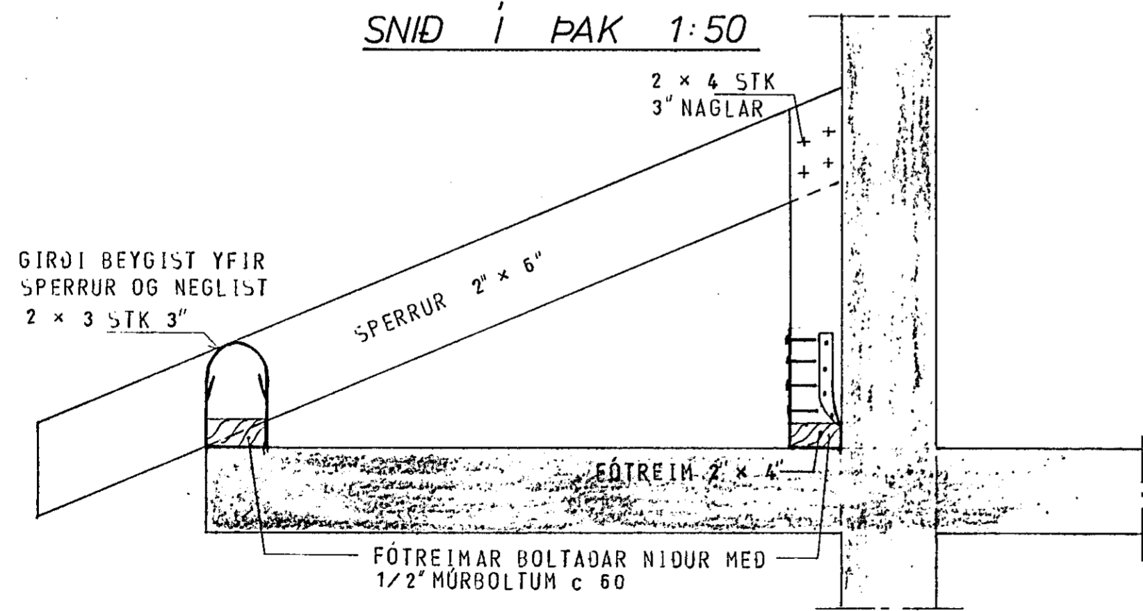
SÉRMÝND 6 1:10
