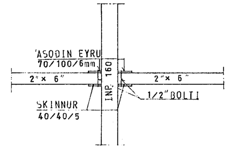
SÉRMÝND 4 1:10
