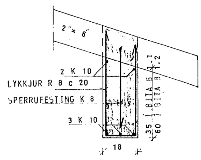
SÉRMÝND 3 1:10
