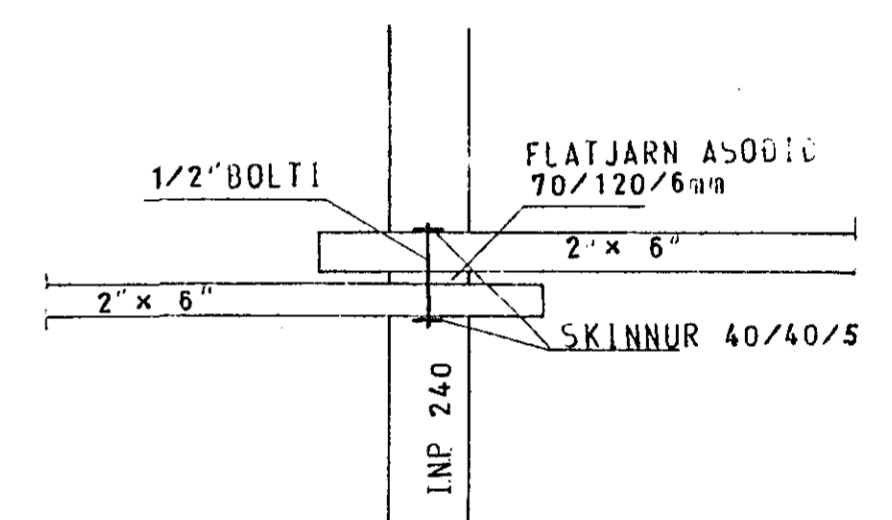
SÉRMÝND 2 1:10
