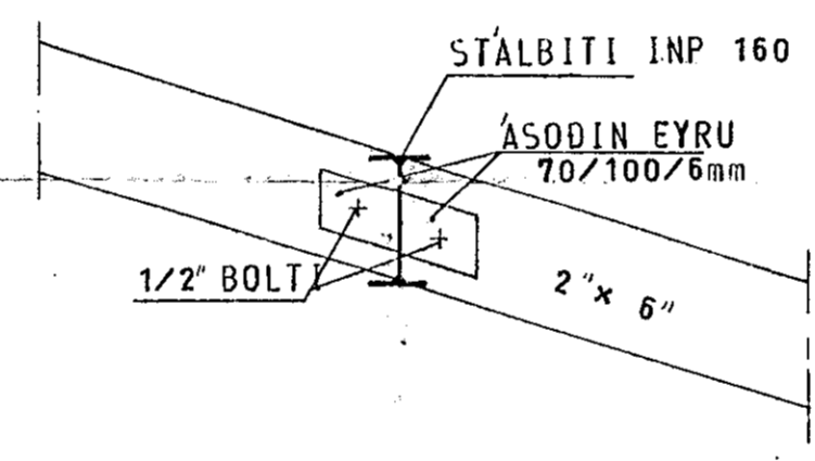
SÉRMÝND 1 1:10
