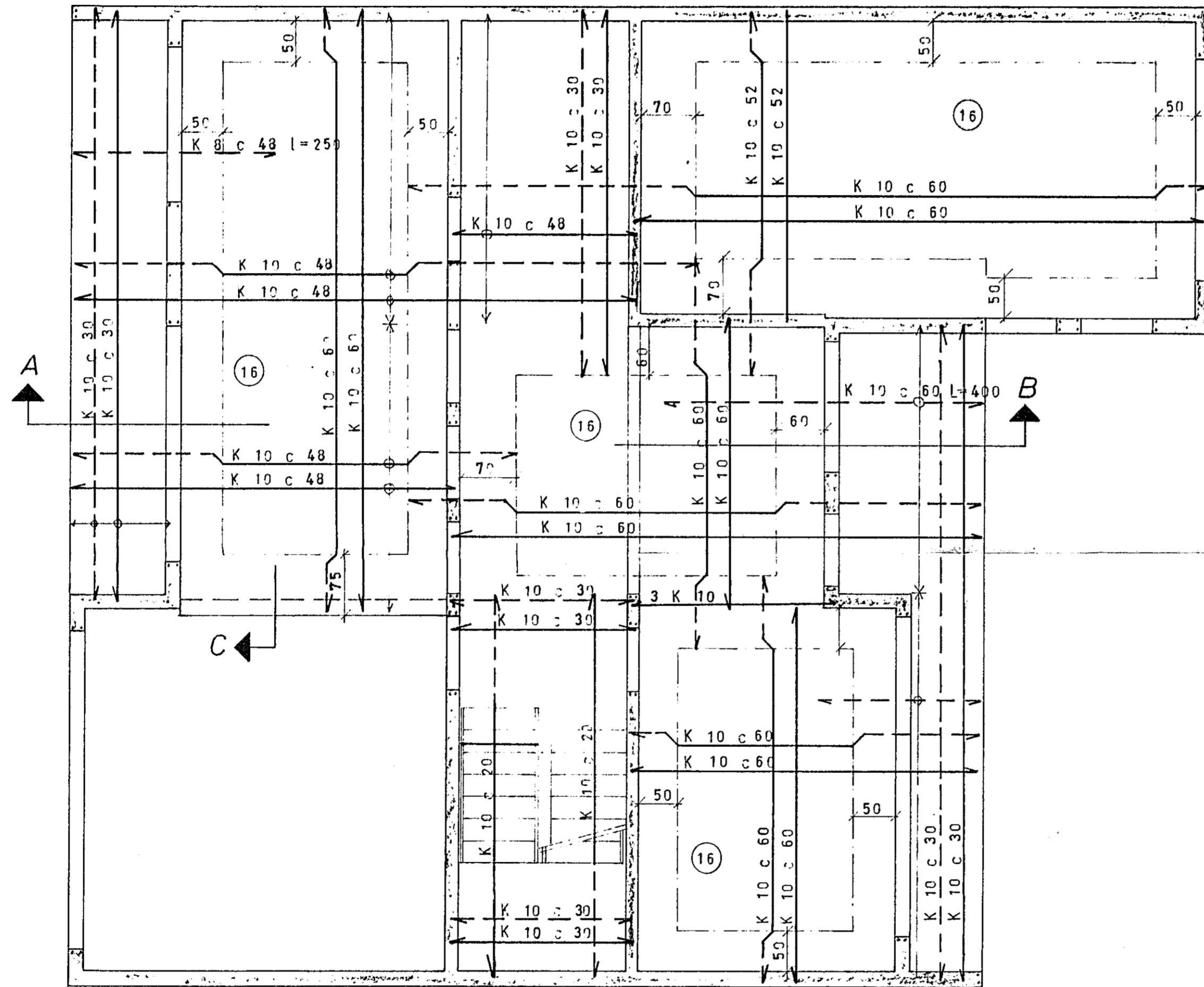
GRUNNMYND — HÆÐAR 1:50
