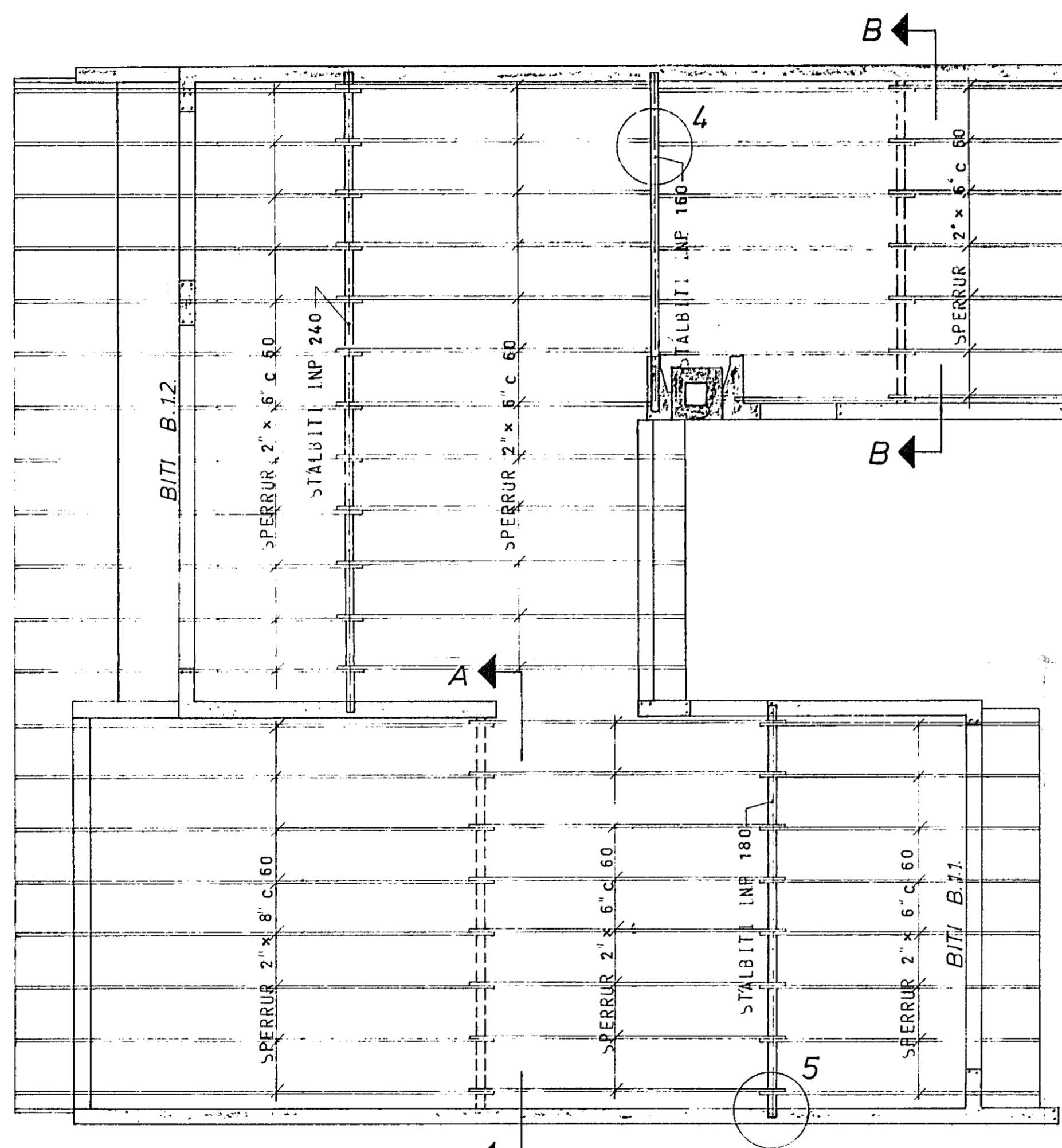
GRUNNMYND - RIS 1:50
