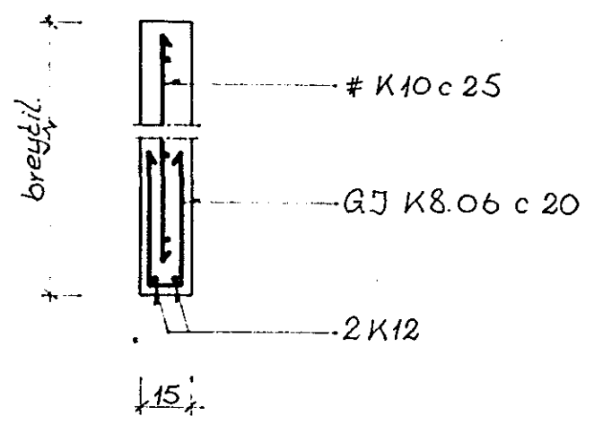
SNID Í B1.10. 1:20
