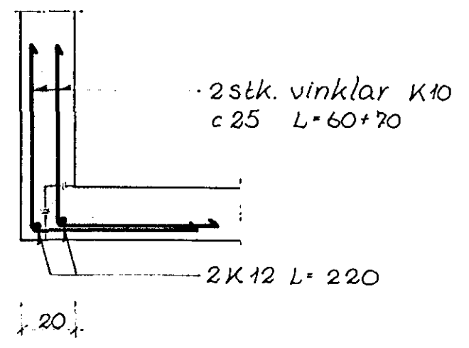
SNID Í B1.11. 1:20
