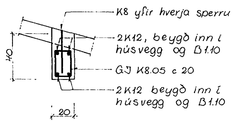
SNID Í B1.11. 1:20
