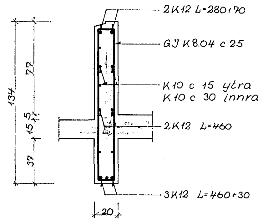
BITI B1.12. 1.stk. 1:20
