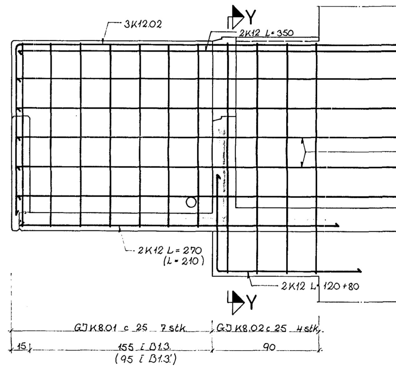
SNID Í B1.4. 1:20
