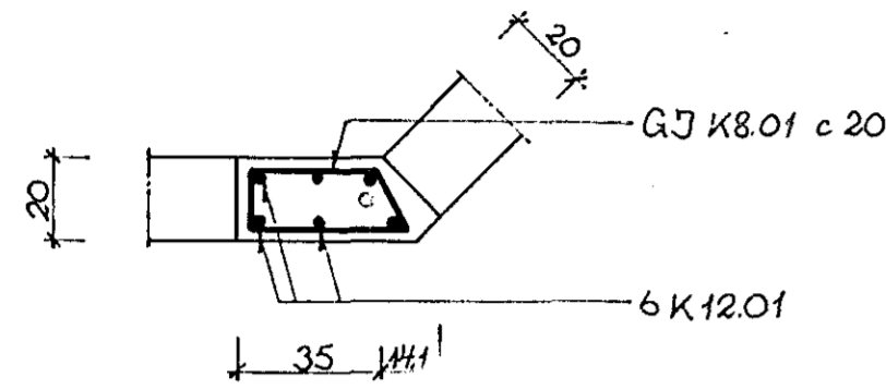
SÚLA S1.1. 1:20 1.stk.
