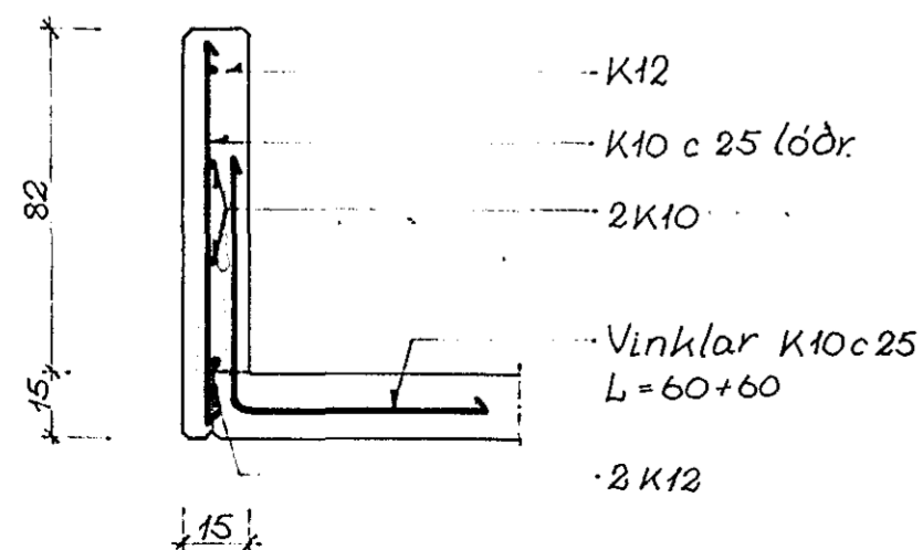
SNID Í B1.1. 4.stk.
