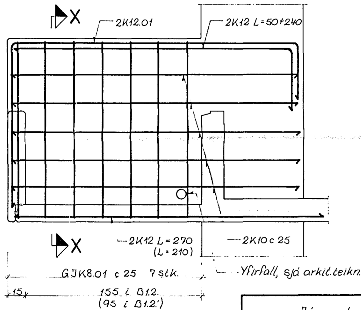
SNID Í B1.1. 4.stk.
