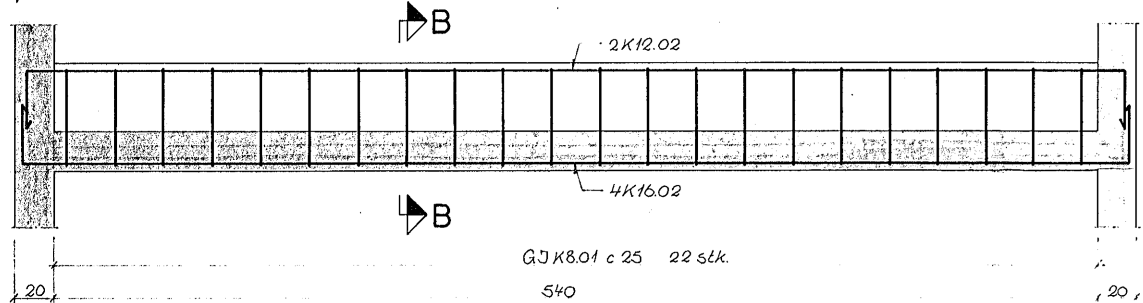
BITI B 3.8. 1:20 1.stk.
