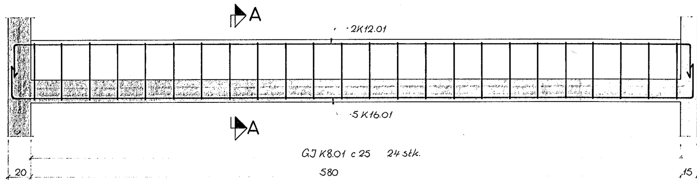
BITI B 3.7. 1:20 2.stk.
