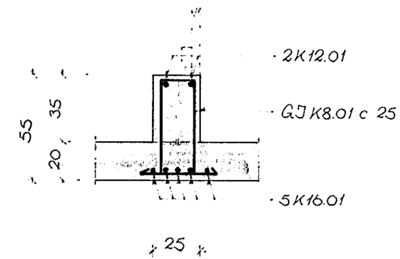
SNID A-A
