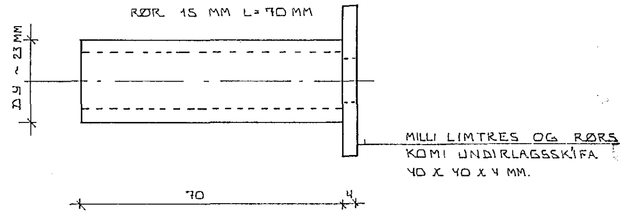
FJARLEGGDARRÖR 1:1
