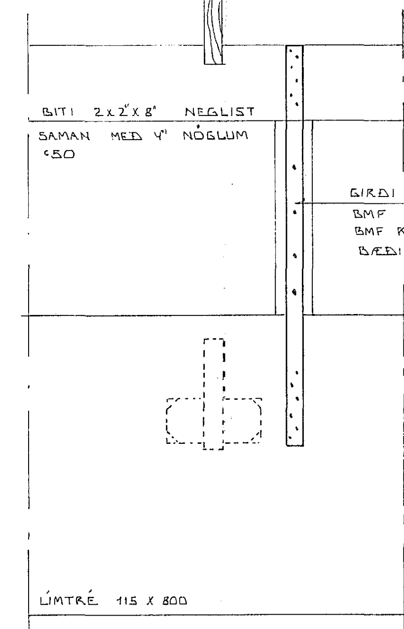
ASÝND B-B 1:10
