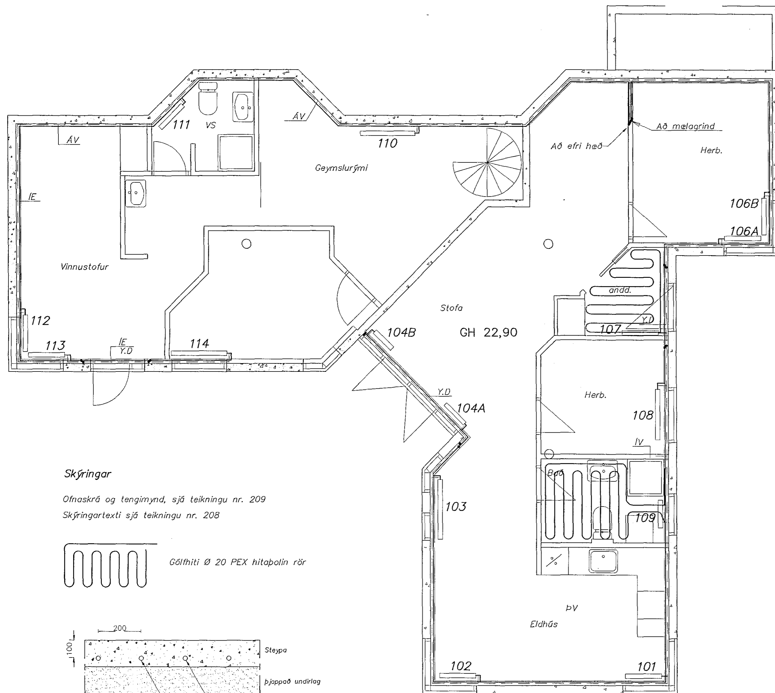
Ø20 PEX rör hitapólin fest við jöfnagrind í steyptri plötu
