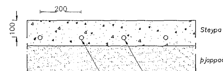
Ø20 PEX rör hitapólin fest við jöfnagrind í steyptri plötu
