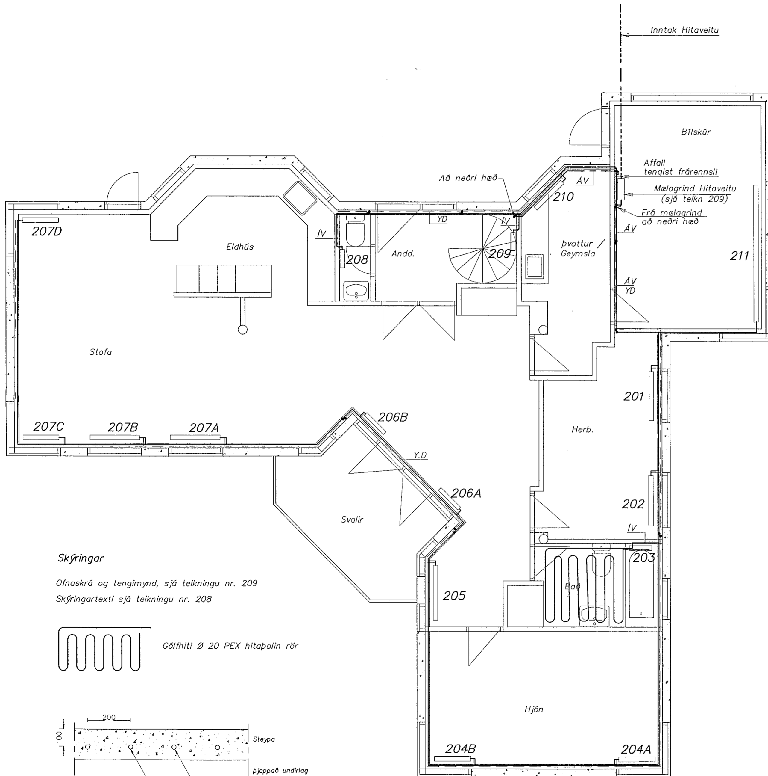
Ø20 PEX rör hitapólin fest við jærnagrind í steyptri plötu
