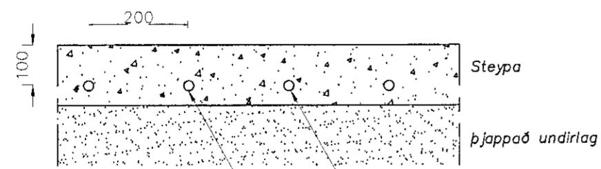
Ø20 PEX rör hitapölin fest við jærnagrind í steyptri plötu
