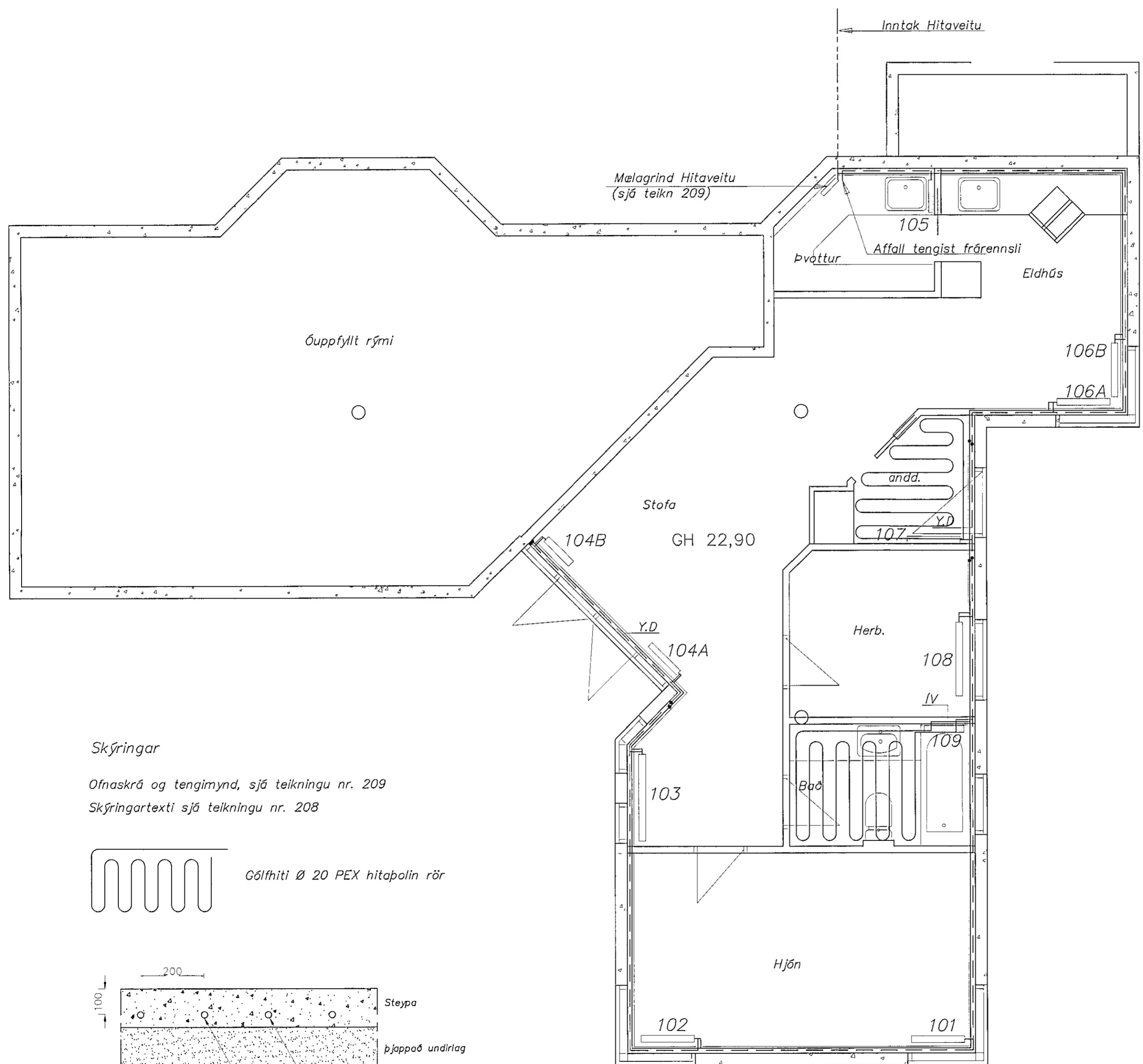
Ø20 PEX rör hitapölin fest við jærnagrind í steyptri plötu
