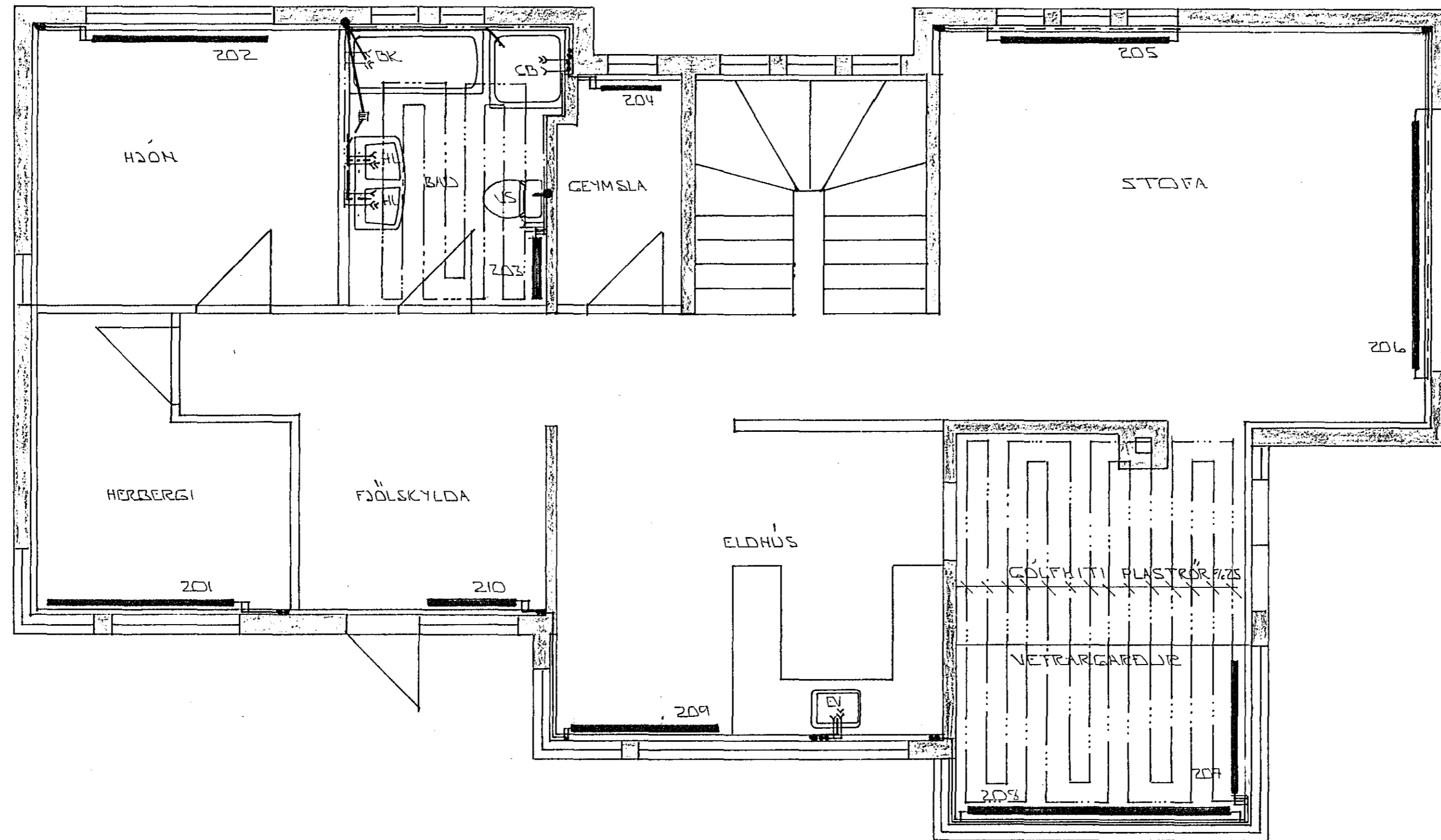
GRUNNMÝND 2. HÆÐ 1:50
