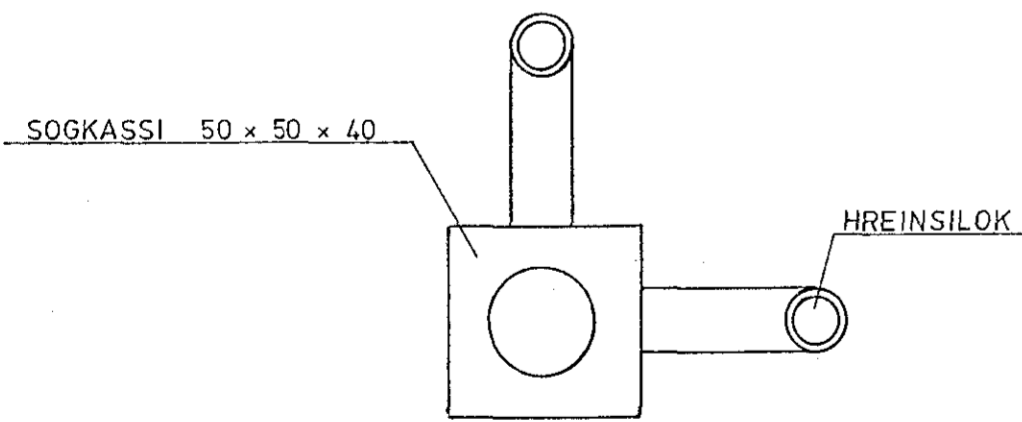
TENING Í SOGKASSA Í ÞAKI 1 : 20
