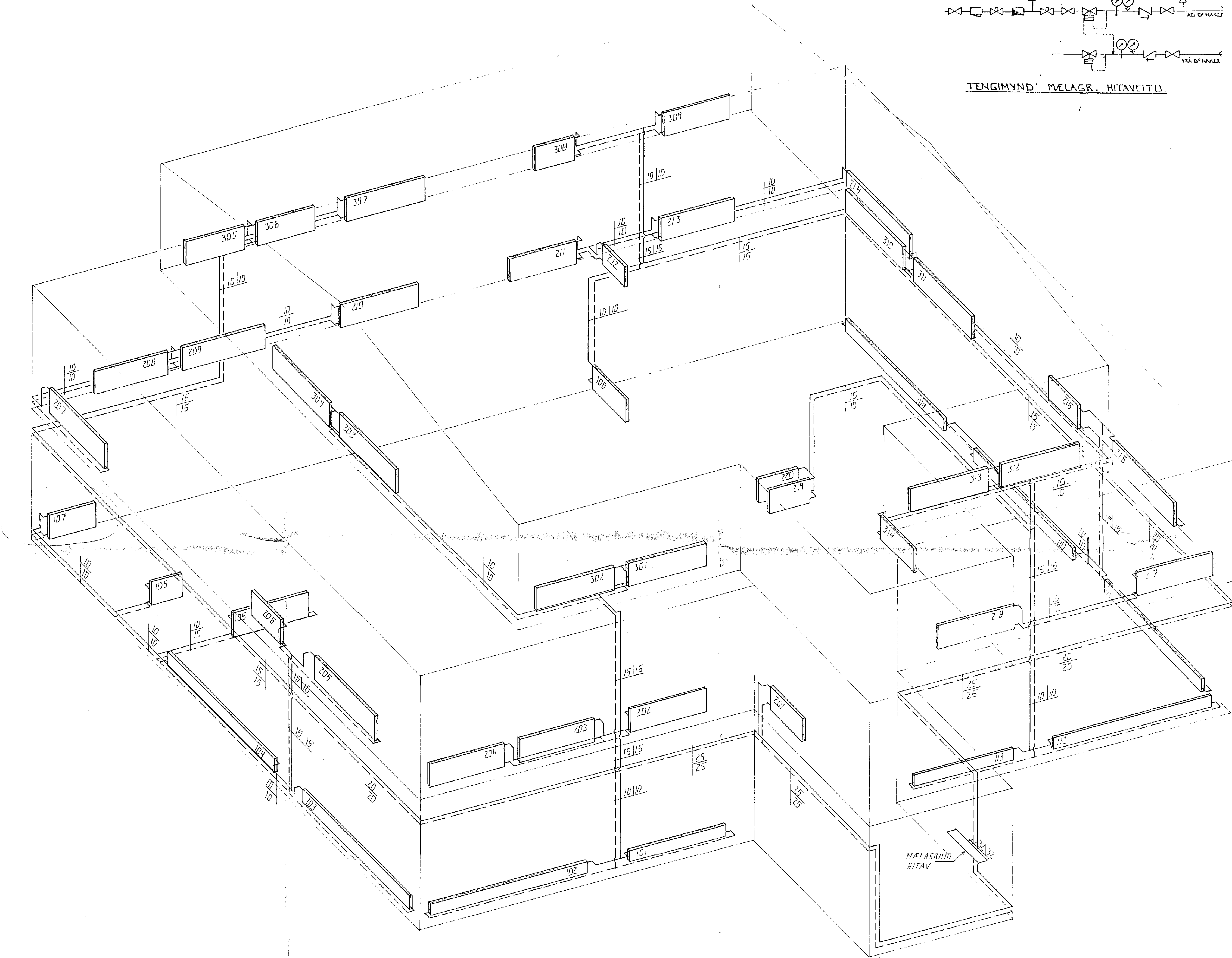
HITALAGNIR RÚMMYND. 1:50
