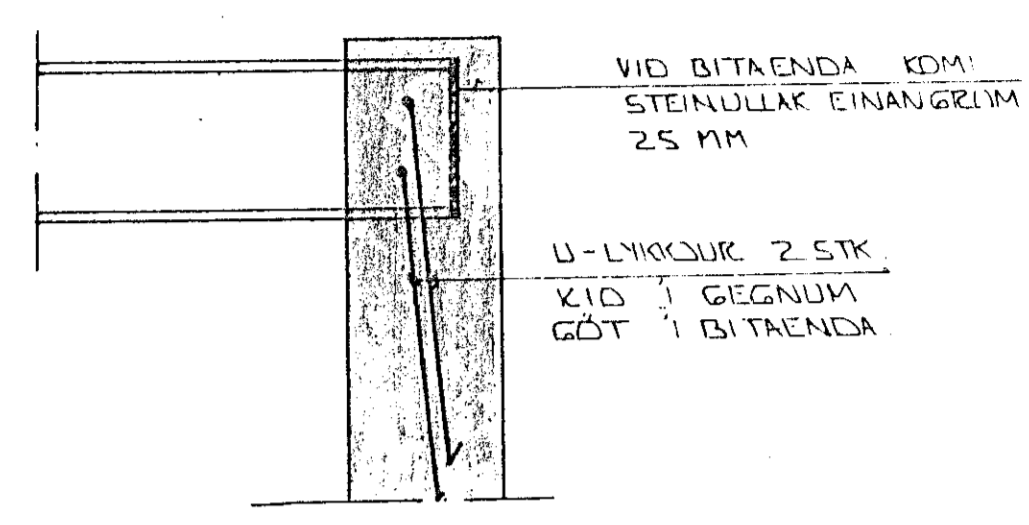
FRÁGANGUR STÁLBITA Í VEGG 1:10 SÉRMYND 14.
