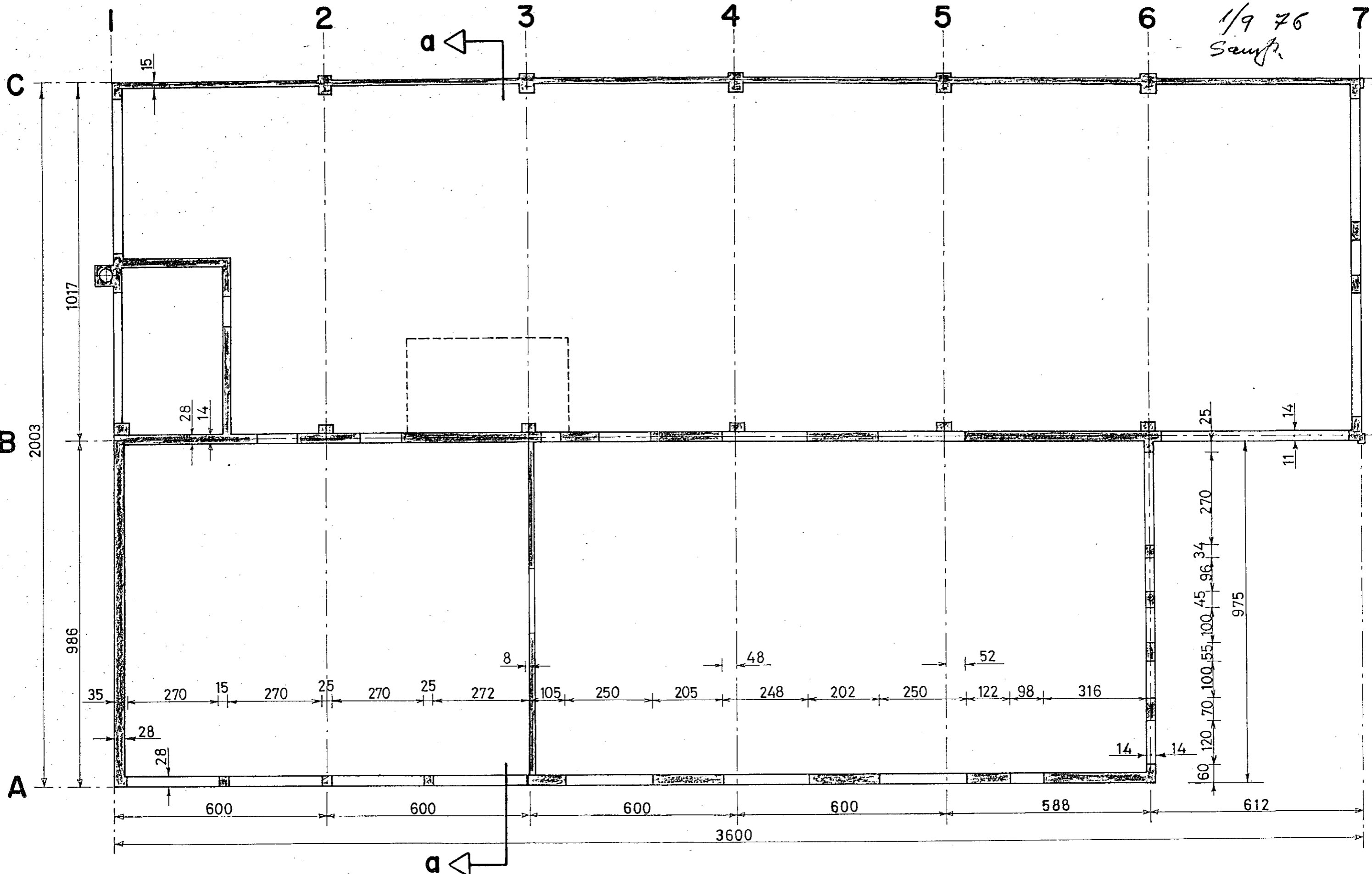
Grunnmynd neðri hæðar 1:100
