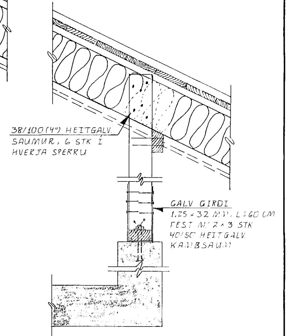
SNID F 12 -F 12 . 1:10
