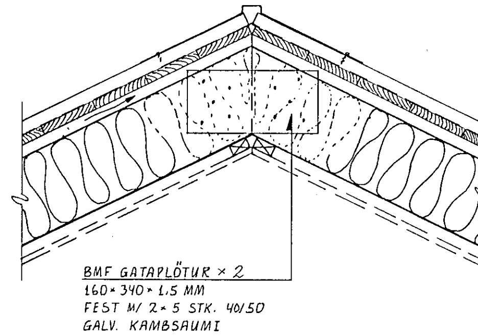
SNID C 12 -C 12 . 1:10
