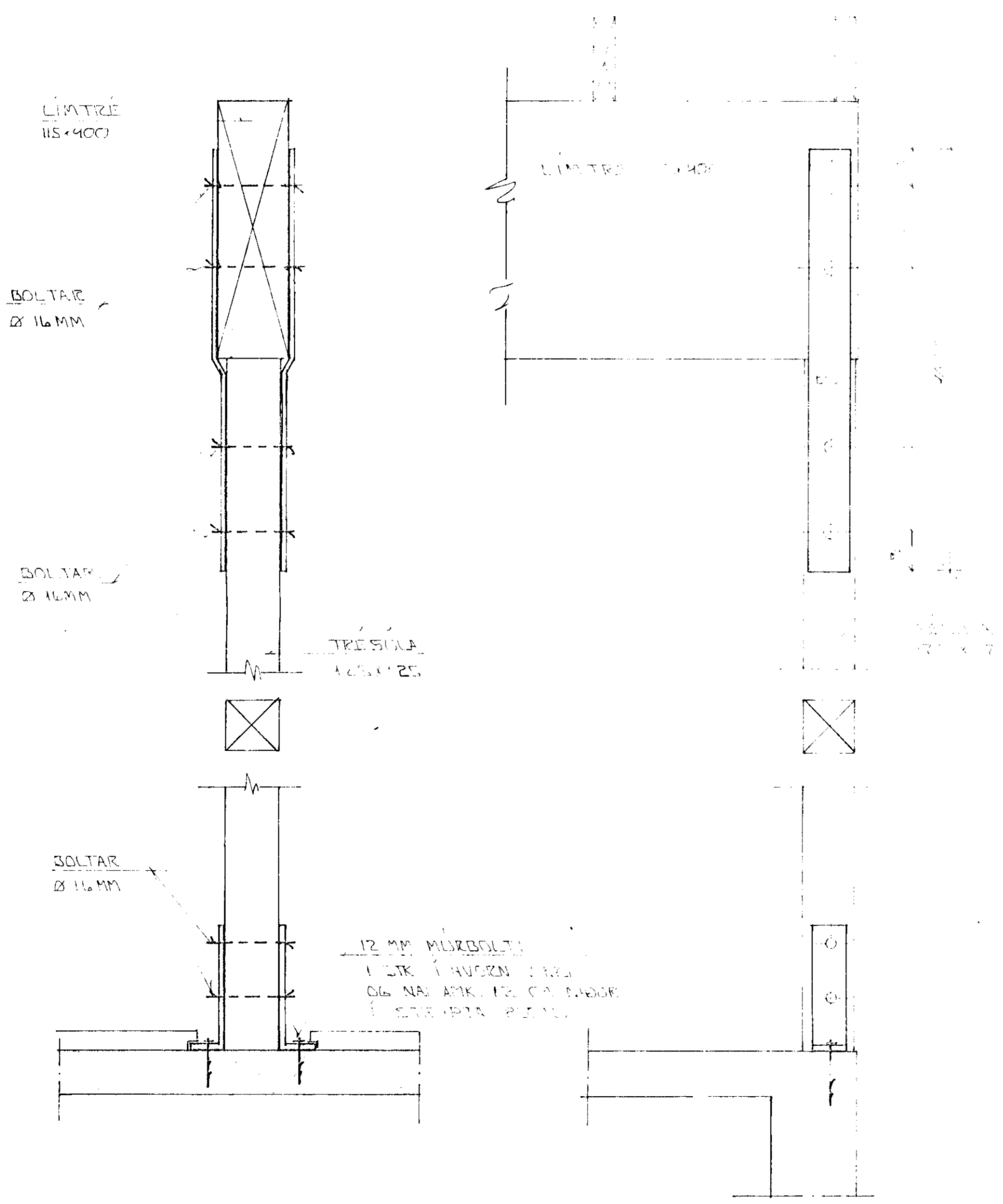
FRÁGANGUR LÍMTRÉSENDA Í VEGG 1:10
