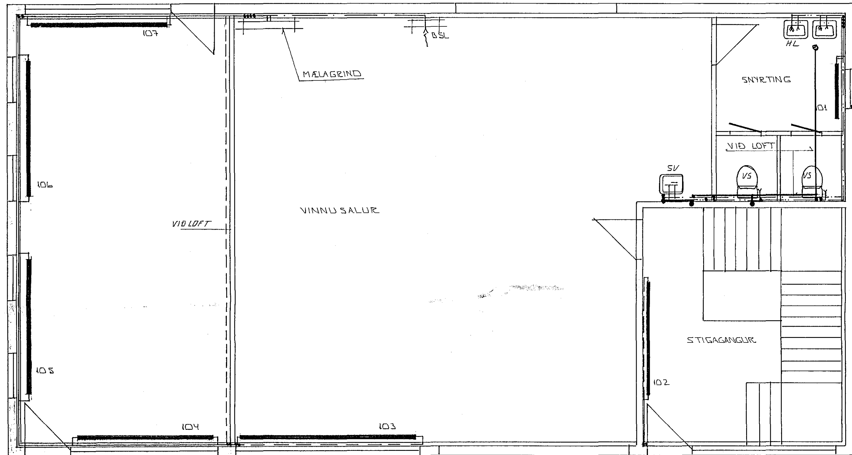
GRUNNMYND I.HÆÐ. 1:50
